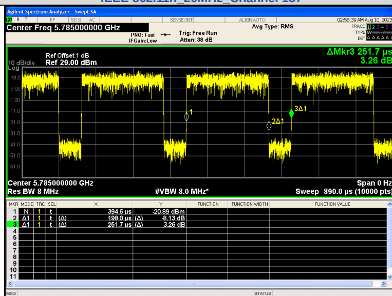
IEEE 802.11n 20MHz Channel 157
