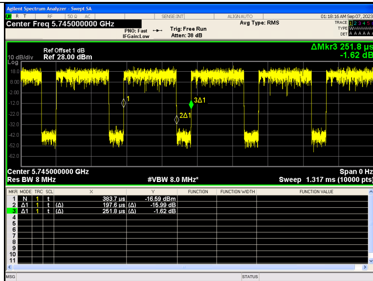
IEEE 802.11n 20MHz Channel 149
