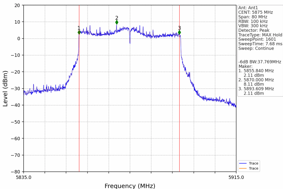
802.11be(EHT40)_MCH_5875MHz_SU_Ant1_NTNV
