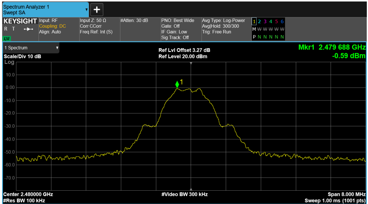
Band Edge NVNT BLE 2480MHz Ant1 Emission
