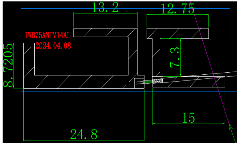
天线尺寸/ANT Size(Unit:mm)
