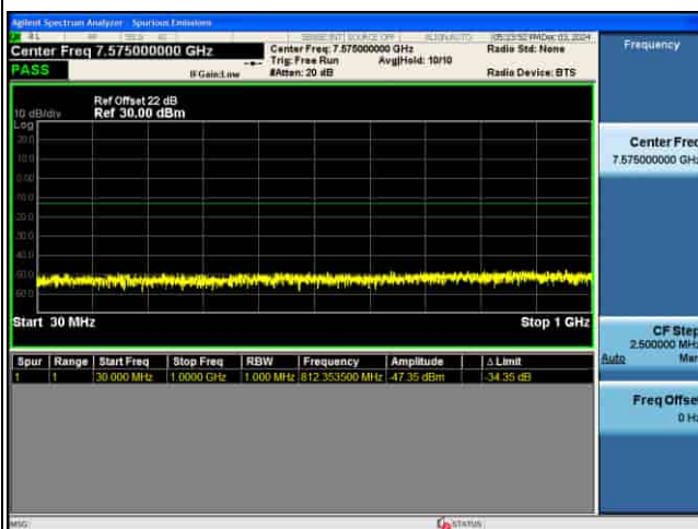
CSE_5G_n77(K)_30KHz_.PI2-BPSK_70M CH634332_1RB@1
