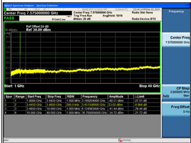
CSE_5G_n77(K)_30KHz_.PI2-BPSK_30M CH633334_1RB@1_
