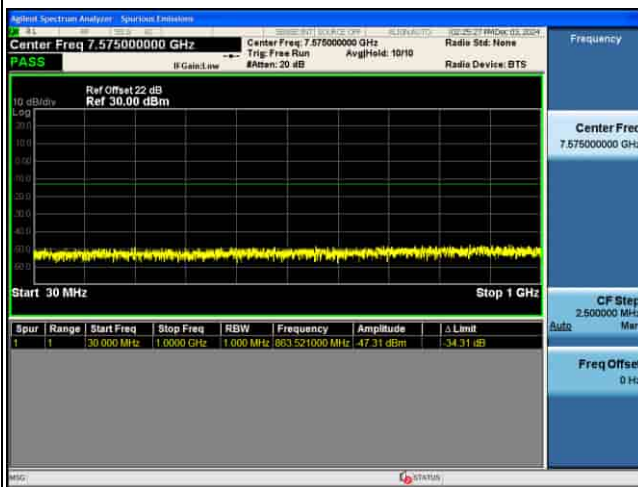
CSE_5G_n77(K)_30KHz_.PI2-BPSK_15M CH633334_1RB@1
