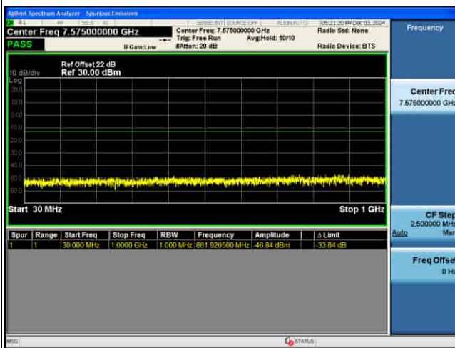
CSE_5G_n77(K)_30KHz_.PI2-BPSK_70M CH633334_1RB@1
