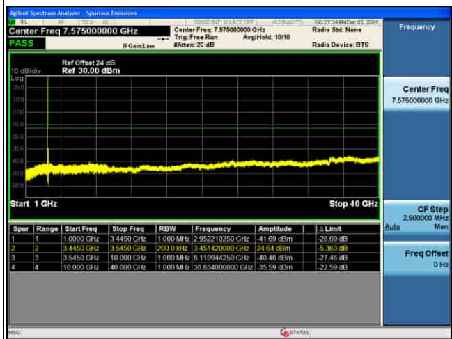
CSE_5G_n77(K)_30KHz_.PI2-BPSK_90M CH633334_1RB@1_
