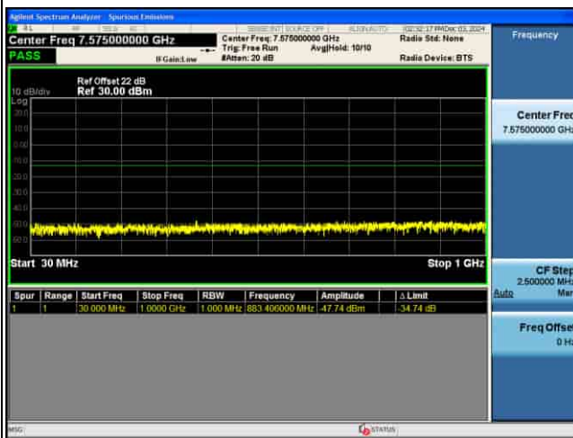
CSE_5G_n77(K)_30KHz_.PI2-BPSK_20M CH633334_1RB@1
