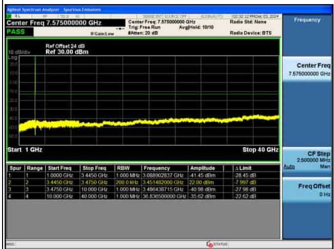
CSE_5G_n77(K)_30KHz_.PI2-BPSK_20M CH633334_1RB@1_
