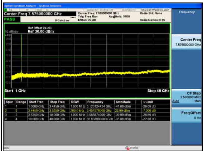
CSE_5G_n77(K)_30KHz_.PI2-BPSK_70M CH633334_1RB@1_
