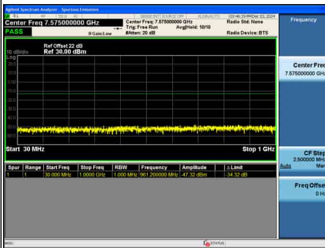
CSE_5G_n77(K)_30KHz_.PI2-BPSK_30M CH633334_1RB@1
