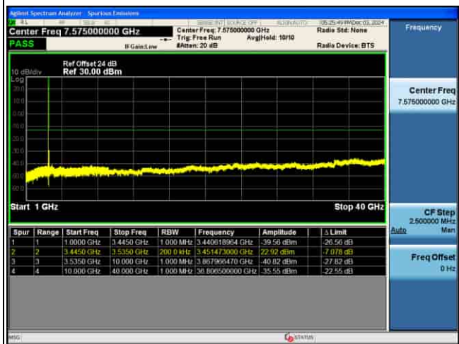
CSE_5G_n77(K)_30KHz_.PI2-BPSK_80M CH633334_1RB@1_
