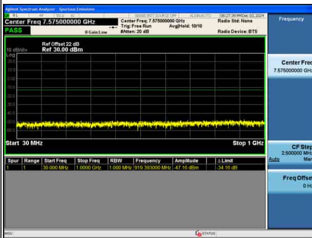
CSE_5G_n77(K)_30KHz_.PI2-BPSK_90M CH633334_1RB@1
