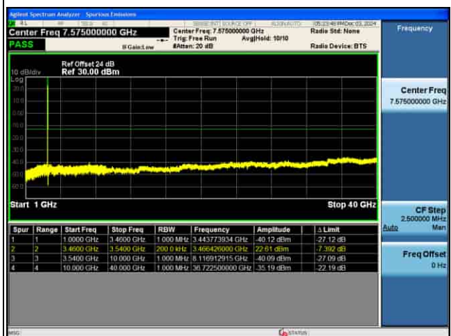
CSE_5G_n77(K)_30KHz_.PI2-BPSK_70M CH634332_1RB@1_
