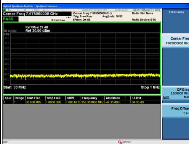
CSE_4G_B42_.QPSK_15M CH43015 1RB@0
