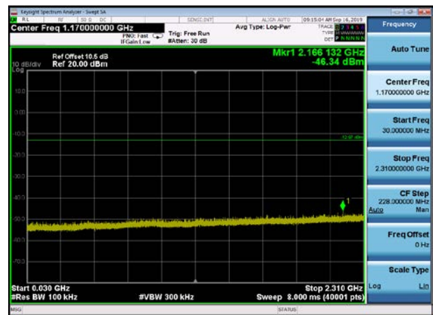
,Plot 3,30MHz~2310MHz-802.11b,2437MHz
