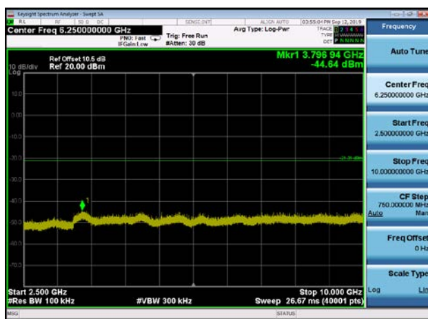
,Plot 4,2500MHz~10000MHz-802.11n(HT40 ) ,2437MHz,Ant0
