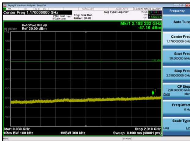
,Plot 3,30MHz~2310MHz-802.11b,2437MHz
