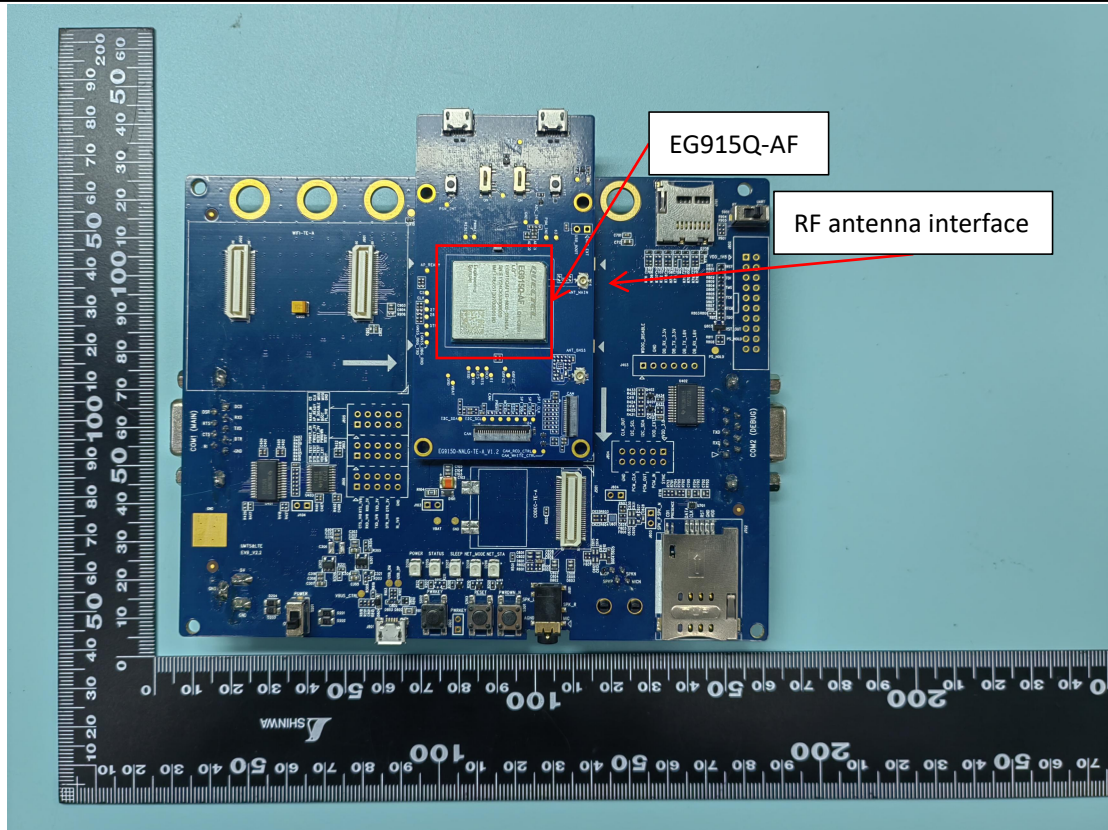
EG915Q-AF + EVB _Top
