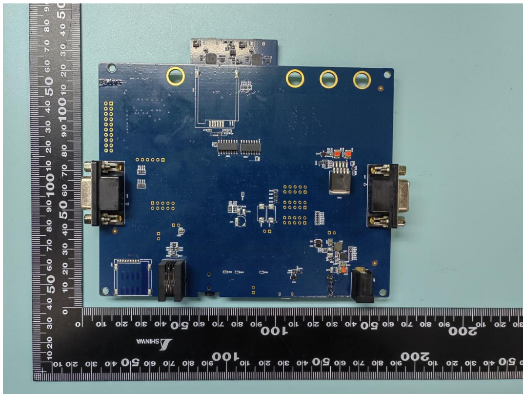
EG915Q-AF + EVB _Bottom
