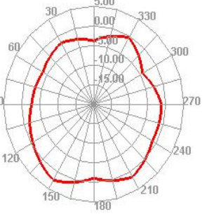
2500.000MHz E2
