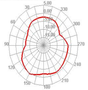
2400.000MHz E2
