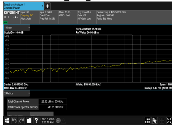
N41(50M)_DFT-s-OFDM_QPSK_Edge_1RB_Left_Low_CH_CHP_PASS
