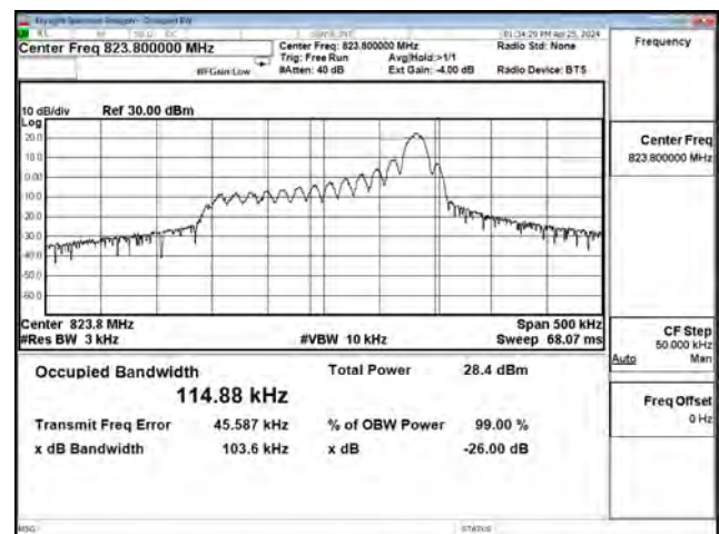
QPSK_CH26788_15k_1RB11
