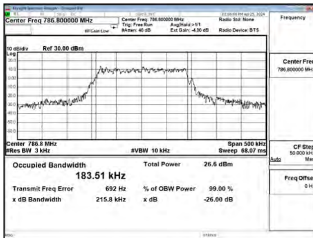
QPSK_CH23278_15k_12RB0
