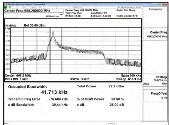
QPSK_CH134180_3.75k_1RB47
