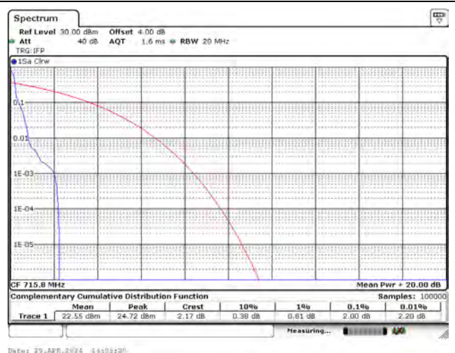
CH23178_3.75k_QPSK_1RB47
