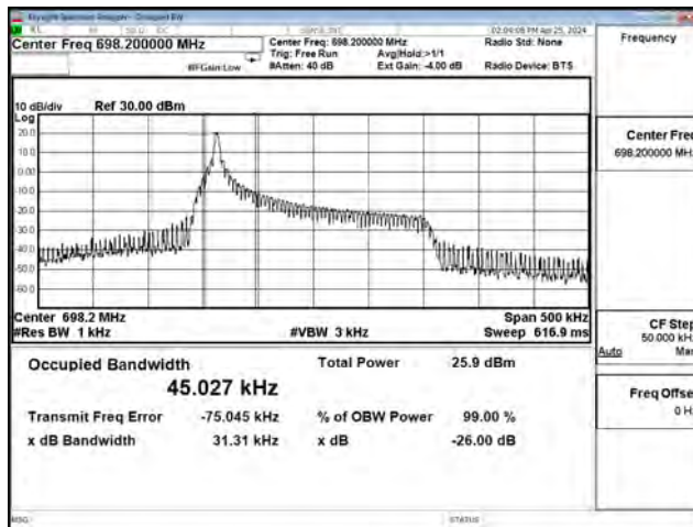
BPSK_CH134180_3.75k_1RB47
