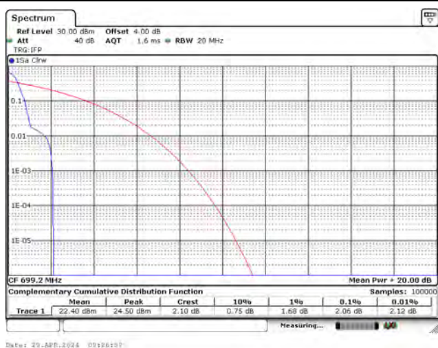
CH23178_15k_BPSK_1RB11
