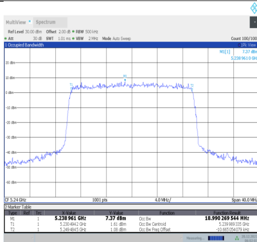
11ax20MIMO-Ant1-5240
