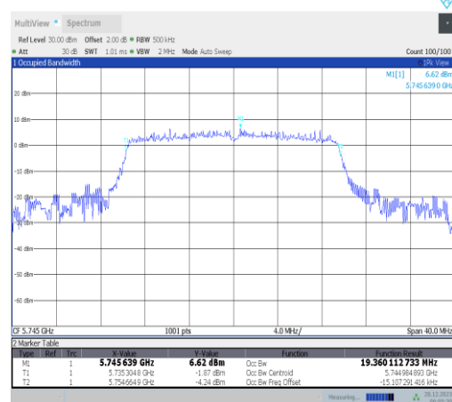
11ax20MIMO-Ant2-5745
