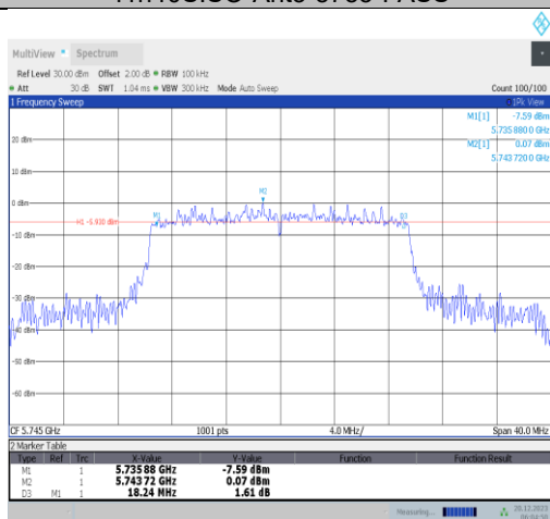
11ax20MIMO-Ant1-5745-PASS
