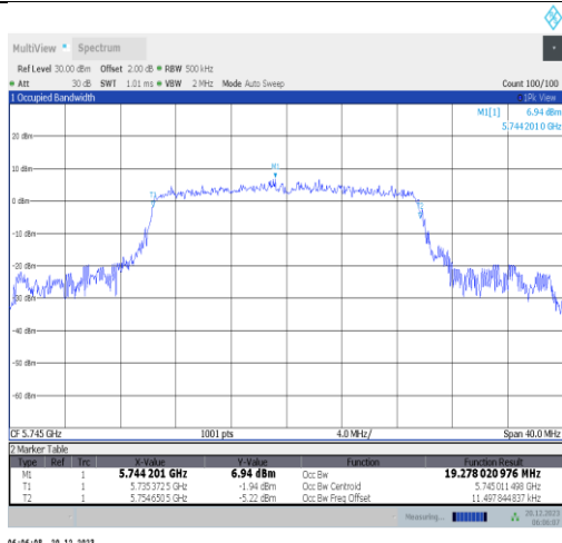
11ax20MIMO-Ant3-5745
