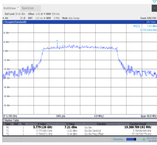
11ax20MIMO-Ant3-5785
