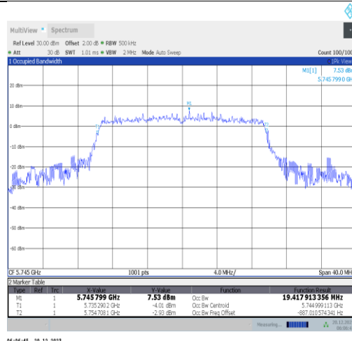
11ax20MIMO-Ant4-5745
