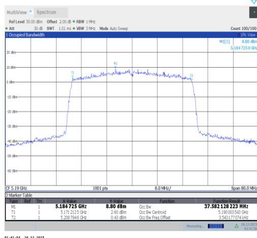
11ax40MIMO-Ant2-5190
