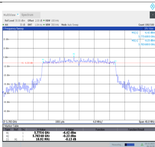
11ax20MIMO-Ant1-5785-PASS
