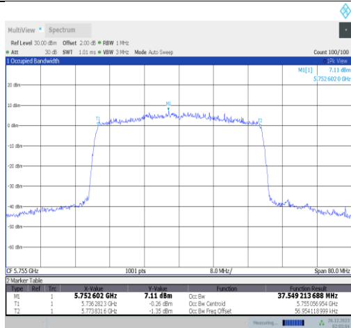
11ax40MIMO-Ant1-5755
