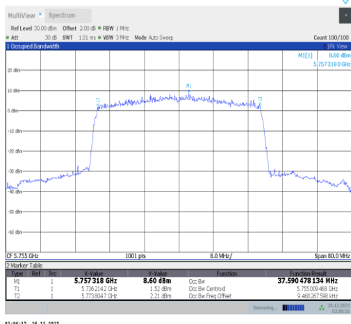
11ax40MIMO-Ant3-5755
