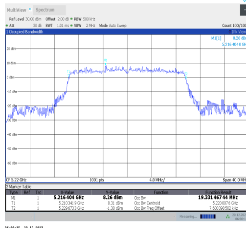
11ax20MIMO-Ant2-5220
