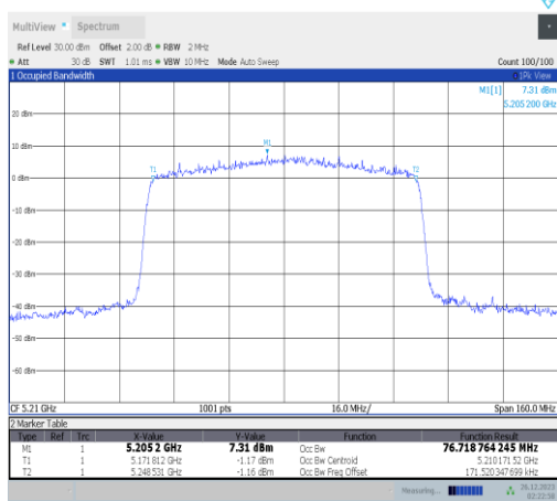
11ax80MIMO-Ant3-5210
