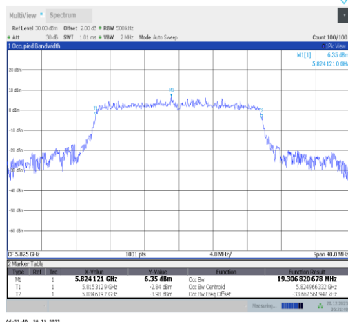
11ax20MIMO-Ant4-5825
