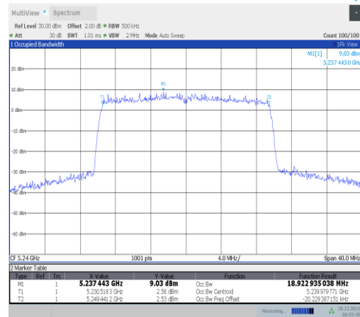
11ax20MIMO-Ant4-5240
