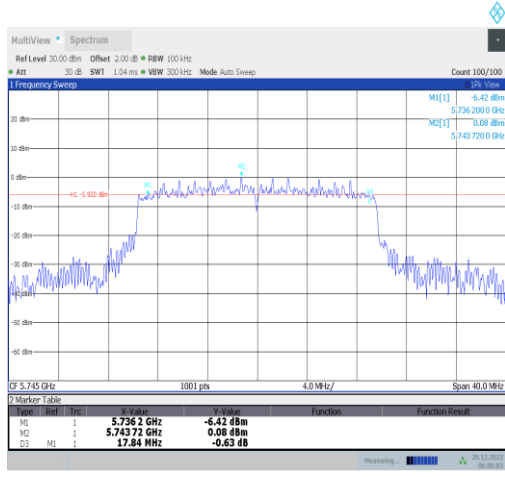
11ax20MIMO-Ant3-5745-PASS
