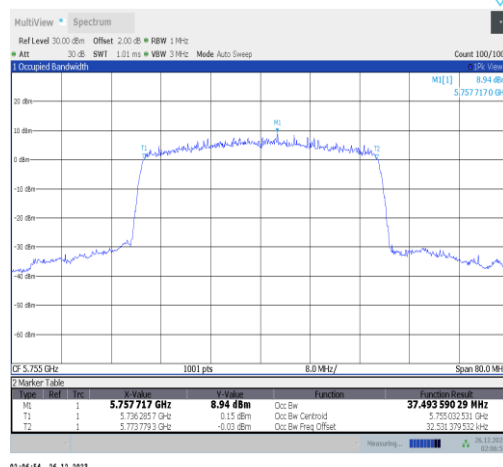
11ax40MIMO-Ant4-5755
