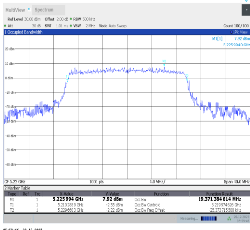
11ax20MIMO-Ant1-5220
