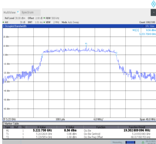
11ax20MIMO-Ant3-5220
