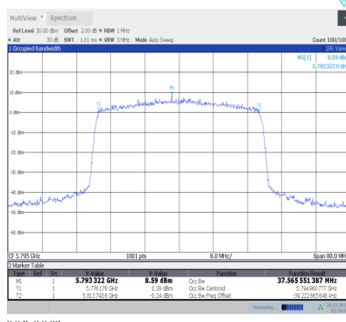
11ax40MIMO-Ant2-5795
