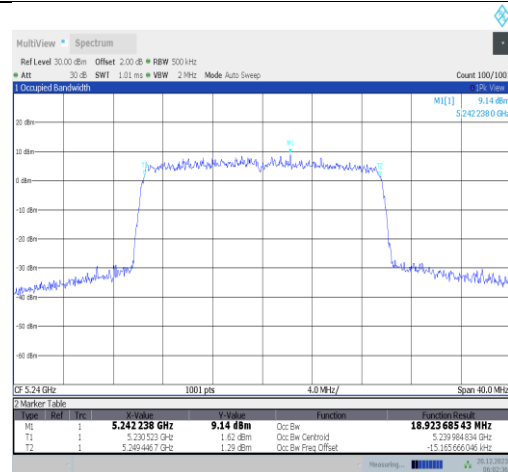
11ax20MIMO-Ant2-5240
