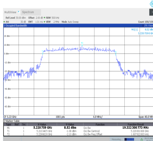
11ax20MIMO-Ant4-5220
