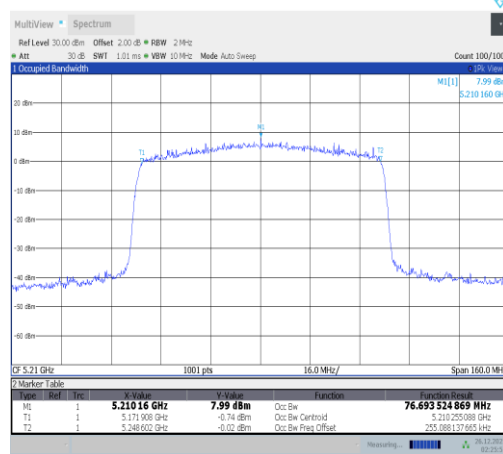
11ax80MIMO-Ant4-5210
