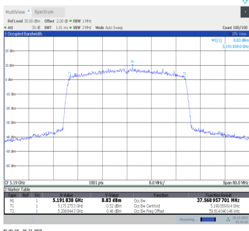
11ax40MIMO-Ant1-5190
