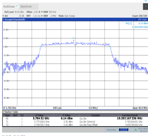
11ax20MIMO-Ant1-5785
