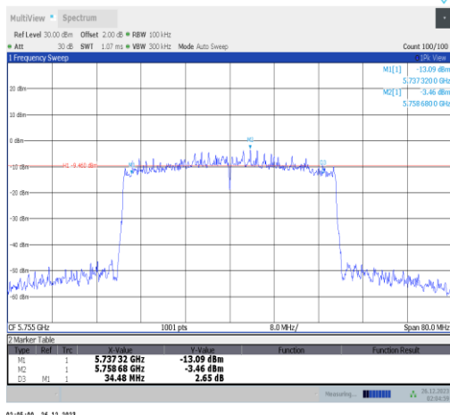
11ax40MIMO-Ant1-5755-PASS
