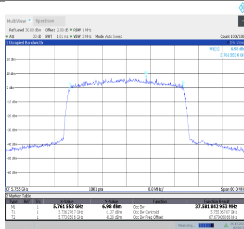
11ax40MIMO-Ant2-5755
