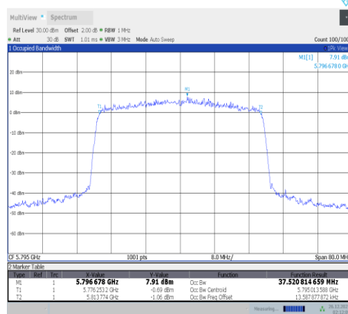
11ax40MIMO-Ant4-5795
