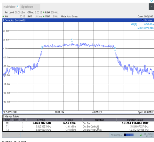
11ax20MIMO-Ant3-5825
