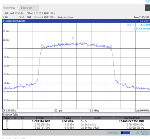
11ax40MIMO-Ant1-5795
