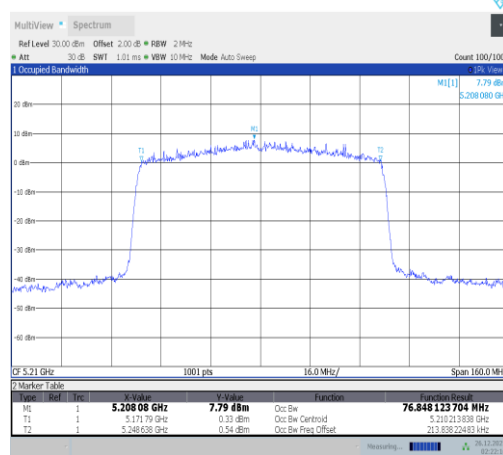
11ax80MIMO-Ant2-5210
