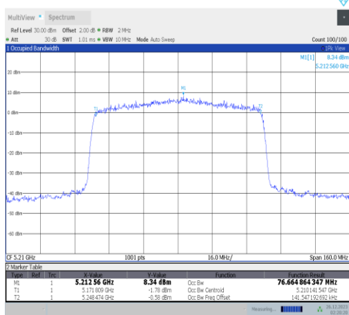
11ax80MIMO-Ant1-5210
