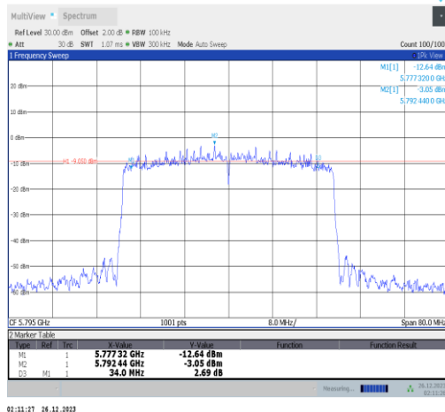
11ax40MIMO-Ant3-5795-PASS
