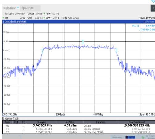
11ax20MIMO-Ant1-5745
