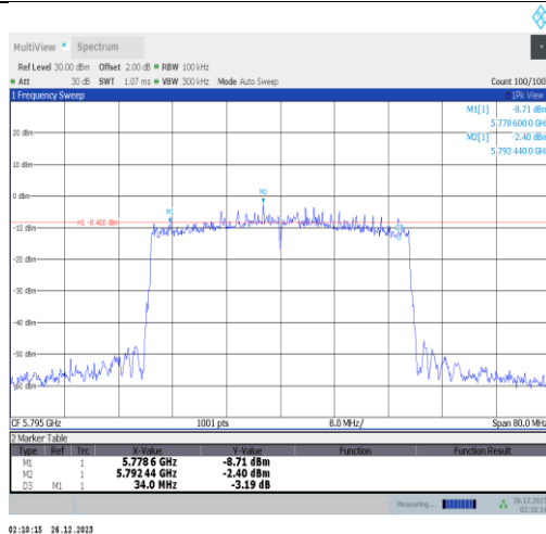
11ax40MIMO-Ant1-5795-PASS
