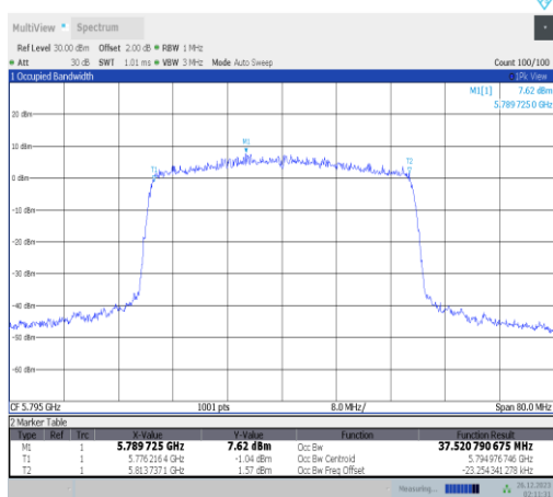
11ax40MIMO-Ant3-5795
