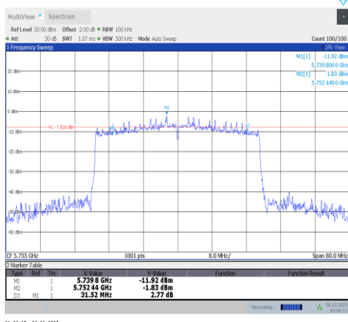
11ax40MIMO-Ant3-5755-PASS
