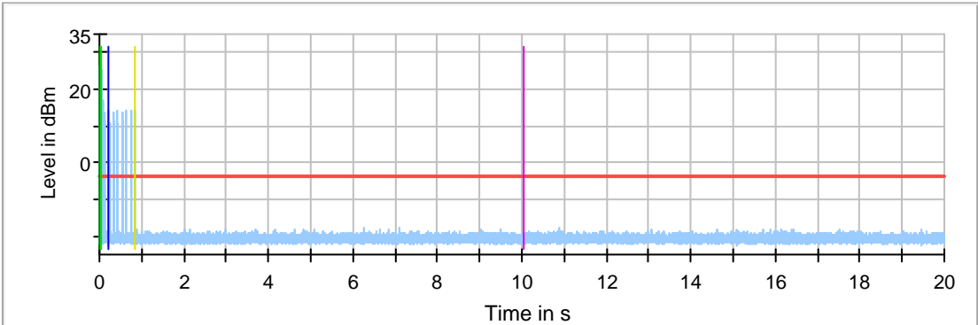
IEEE 802.11n HT40 5270MHz
