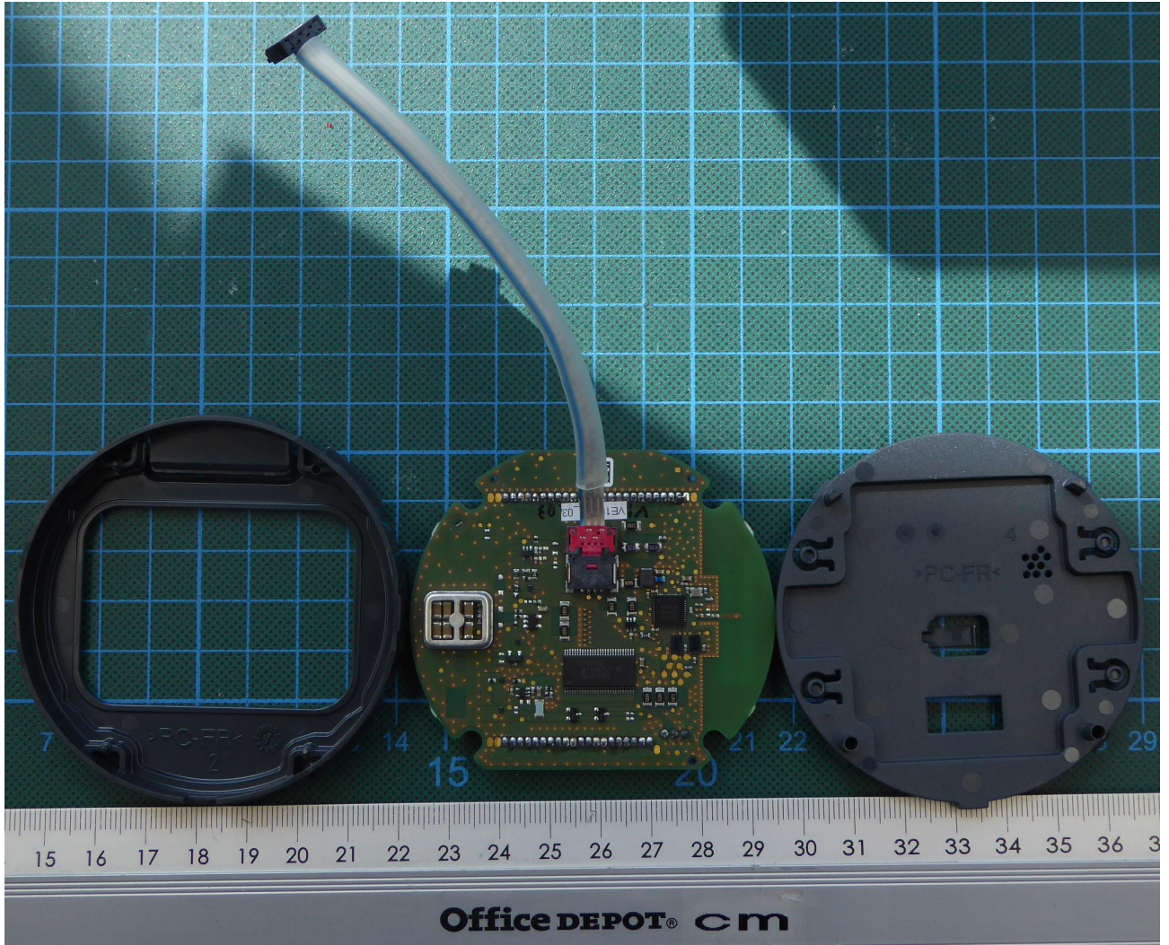
VE_101_A_03 – EUT open
