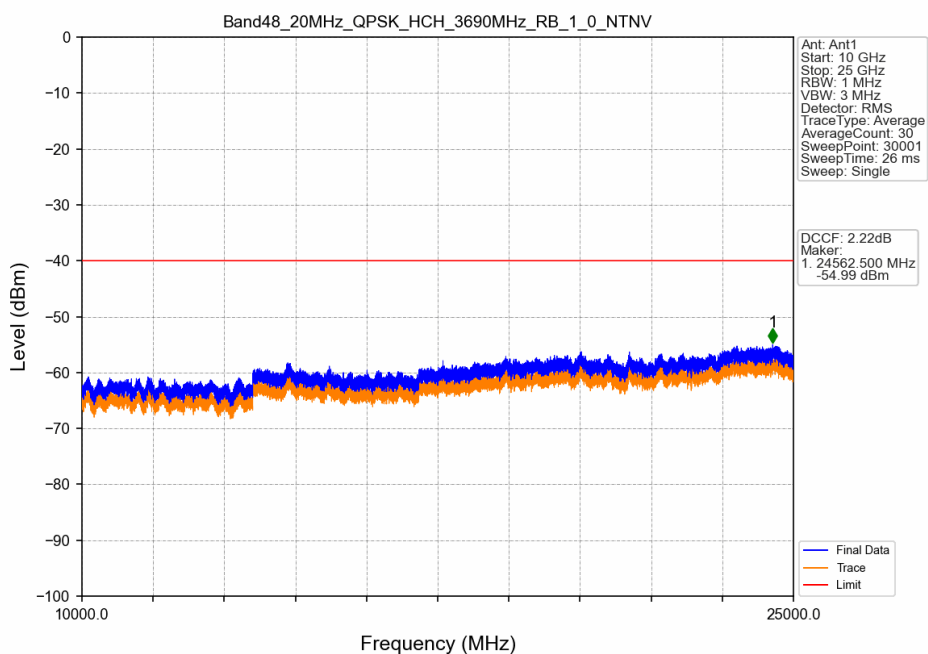
Band48_20MHz_QPSK_HCH_3690MHz_RB_1_0_NTNV
