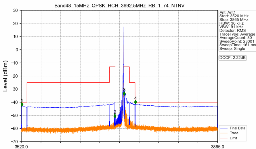
Band48_15MHz_QPSK_HCH_3692.5MHz_RB_1_74_NTNV
