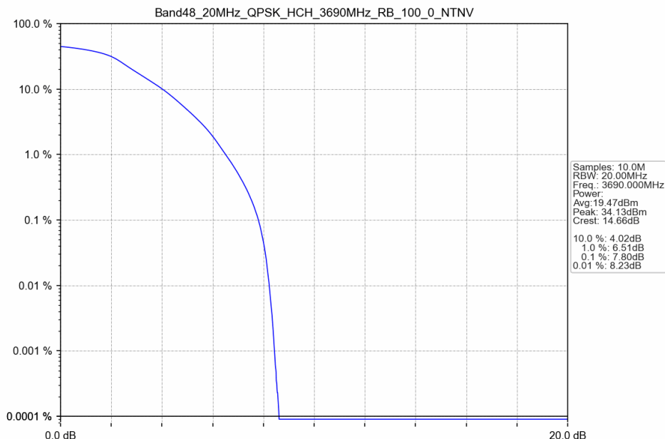
Band48_20MHz_QPSK_HCH_3690MHz_RB_100_0_NTNV
