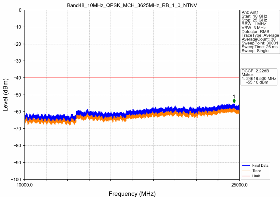
Band48_10MHz_QPSK_MCH_3625MHz_RB_1_0_NTNV
