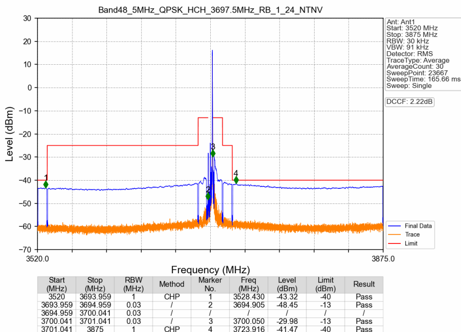
Band48_5MHz_QPSK_HCH_3697.5MHz_RB_1_24_NTNV
