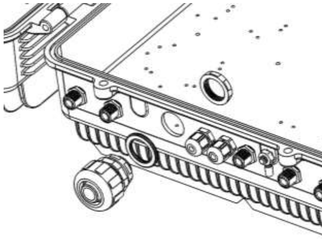
A - Remove the conduit connector
