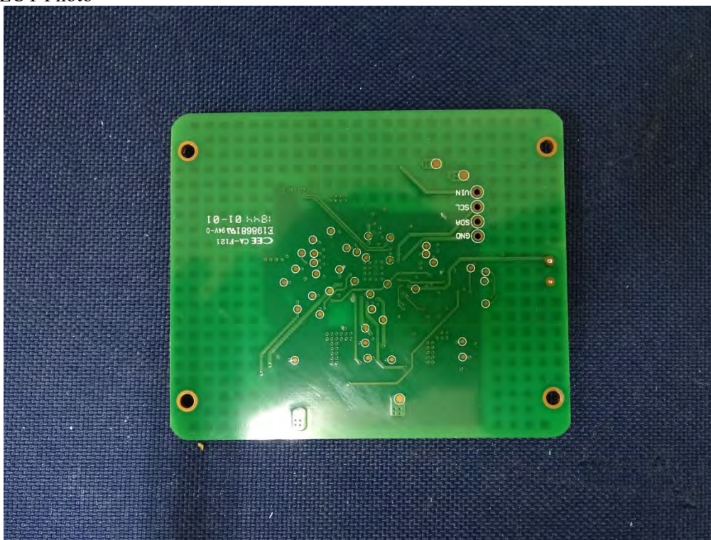
(47) EUT Photo
