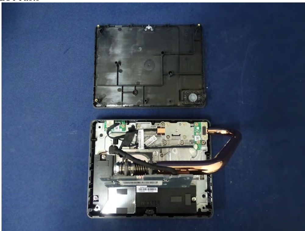
(31) EUT Photo
