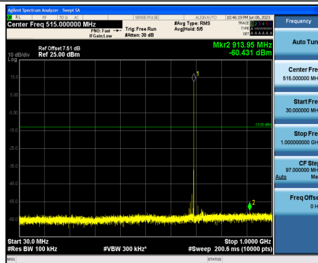
Band12-5MHz-QPSK-23035-1-0-Low-30-1000--60.43-PASS
