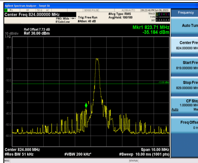
Band5-3MHz-16QAM-20415-1-0-Low--35.18-PASS
