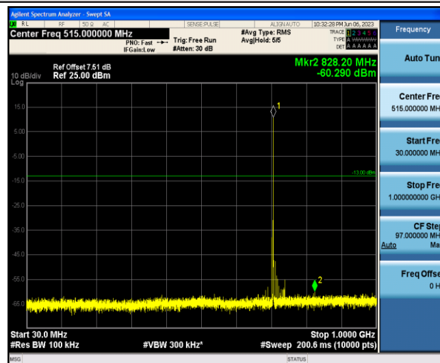
Band12-3MHz-16QAM-23165-1-0-Low-30-1000--60.29-PASS
