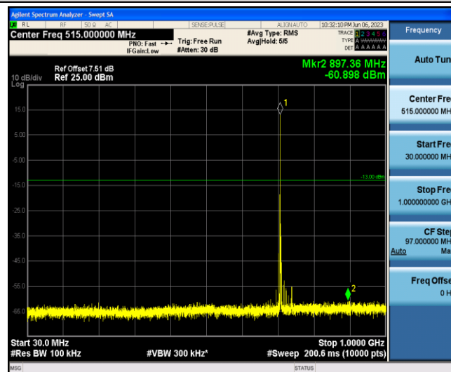
Band12-3MHz-QPSK-23165-1-0-Low-30-1000--60.9-PASS
