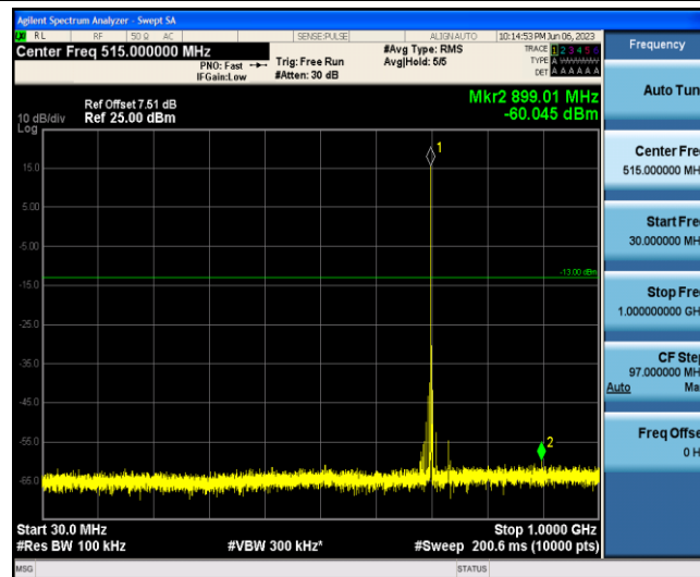
Band12-1.4MHz-16QAM-23095-1-0-Low-30-1000--60.05-PASS
