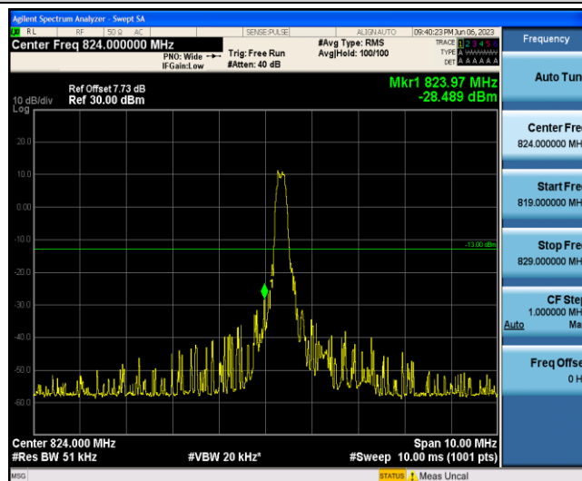
Band5-5MHz-16QAM-20425-1-0-Low--28.49-PASS
