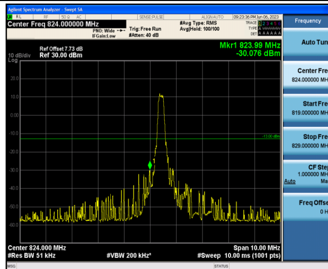
Band5-3MHz-QPSK-20415-1-0-Low--30.08-PASS
