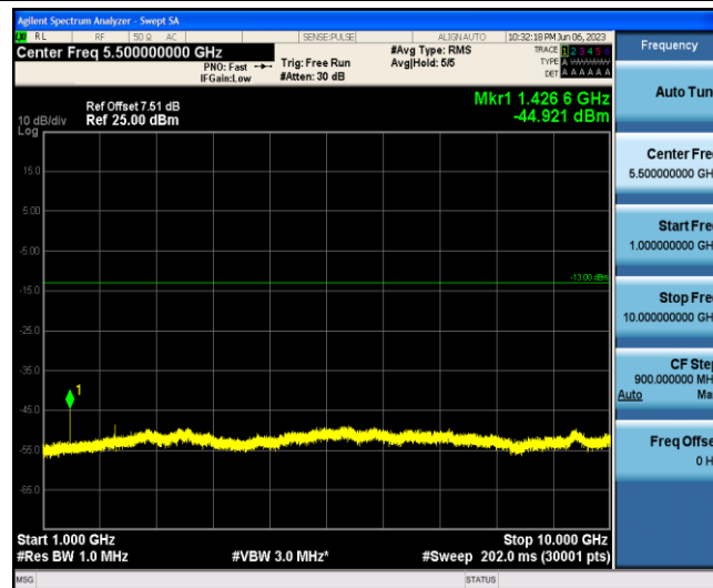
Band12-3MHz-QPSK-23165-1-0-Low-1000-10000--44.92-PASS
