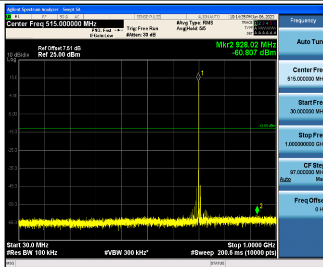
Band12-1.4MHz-QPSK-23095-1-0-Low-30-1000--60.81-PASS
