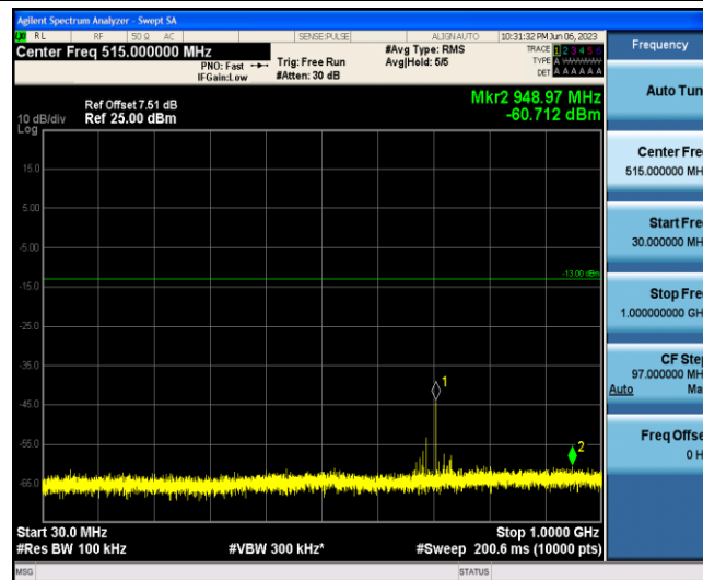
Band12-3MHz-QPSK-23095-1-0-Low-30-1000--60.71-PASS
