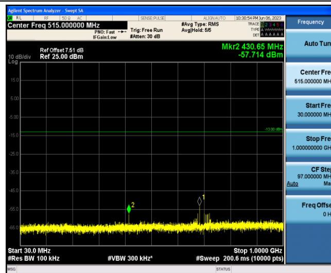
Band12-3MHz-QPSK-23025-1-0-Low-30-1000--57.71-PASS
