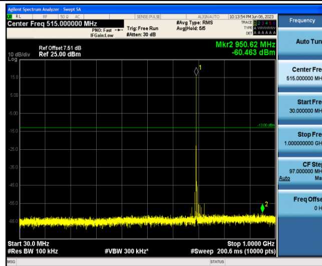
Band12-1.4MHz-QPSK-23017-1-0-Low-30-1000--60.46-PASS
