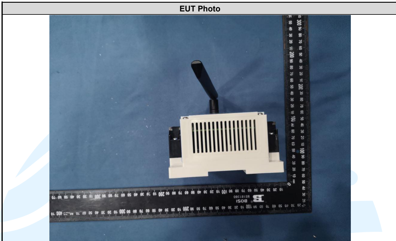
EUT Photo-Ports
