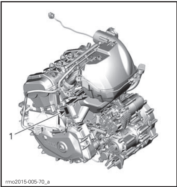
TYPICAL 1. EIN (Engine Identification Number) location
