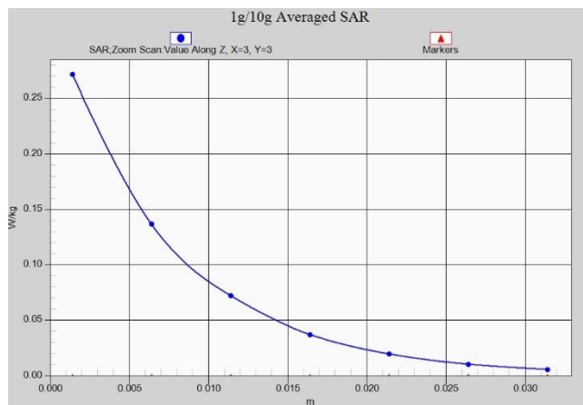
N38 Body 15mm ANT1
