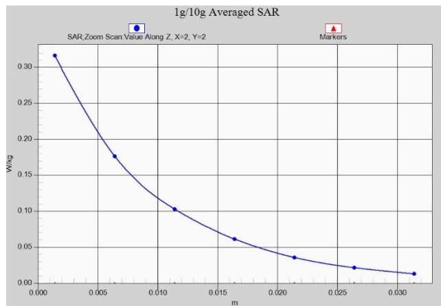
LTE Band25 Body 10mm ANT1
