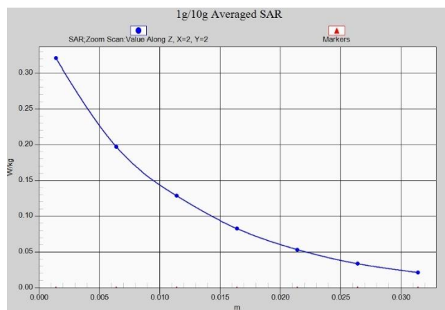
N66 Body 15mm ANT1
