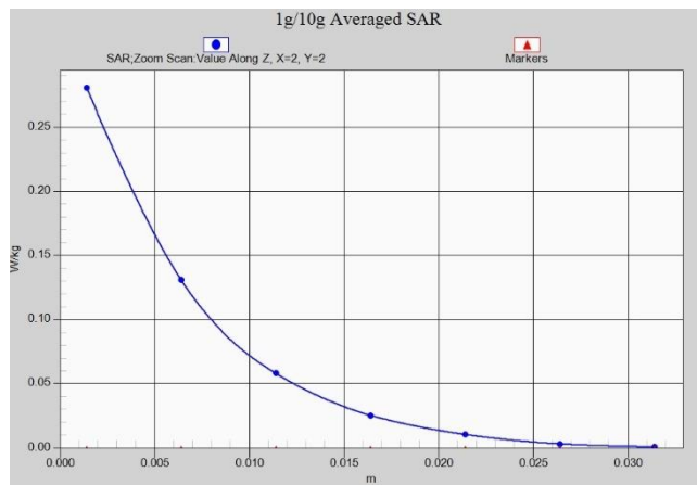
N38 Body 10mm ANT1
