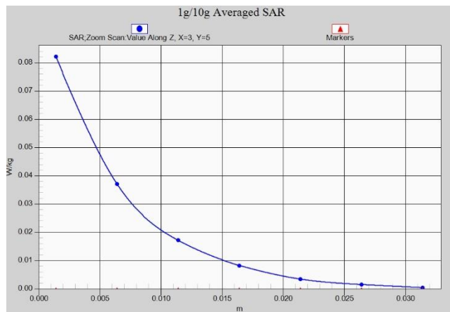
LTE Band41 PC3 Body 10mm ANT1
