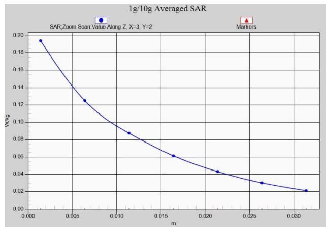
LTE Band25 Head ANT1
