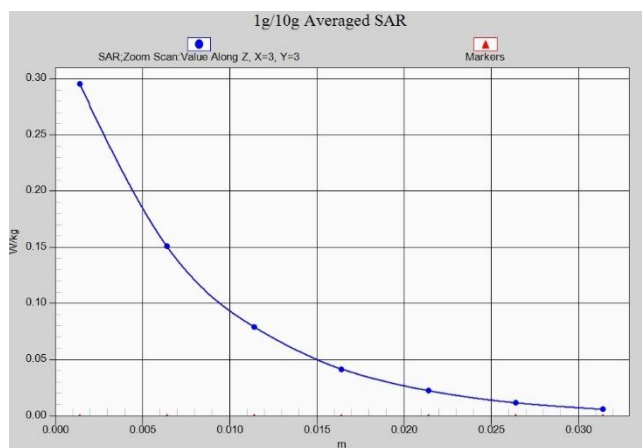
N7 Body 15mm ANT1
