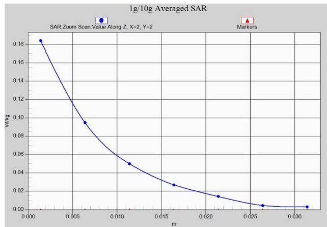
N38 Head ANT1
