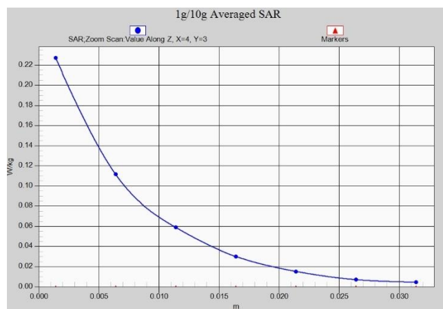
N41 Body 15mm ANT1
