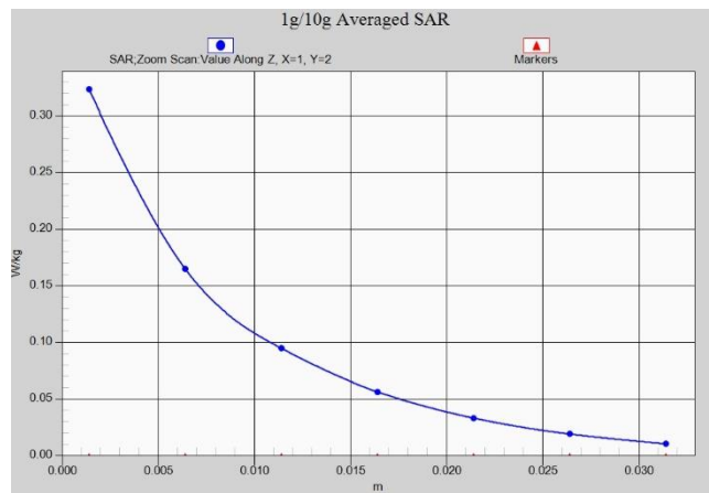
N66 Body 10mm ANT1
