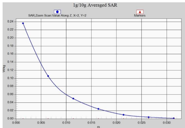
N7 Body 10mm ANT1
