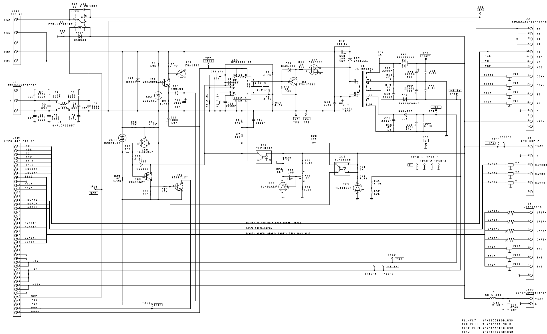
【図115 CBD - 1596 電源回路接続図】
