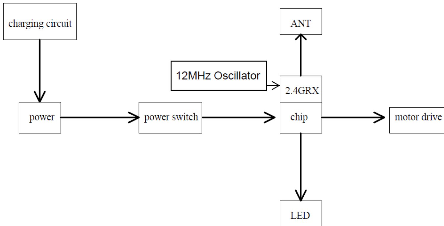
66804RXV12-block diagram
