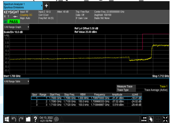
B66(15.0M) 16QAM 75@0 132047 CH
