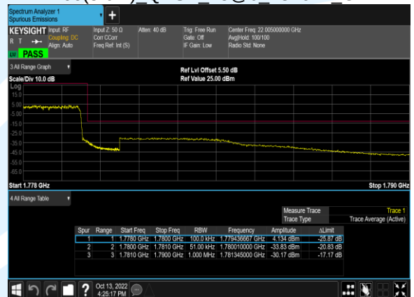
B66(5.0M) 16QAM 25@0 132647 CH
