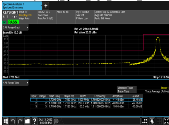
B66(20.0M) 16QAM 1@0 132072 CH
