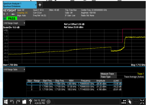
B66(5.0M) 16QAM 25@0 131997 CH
