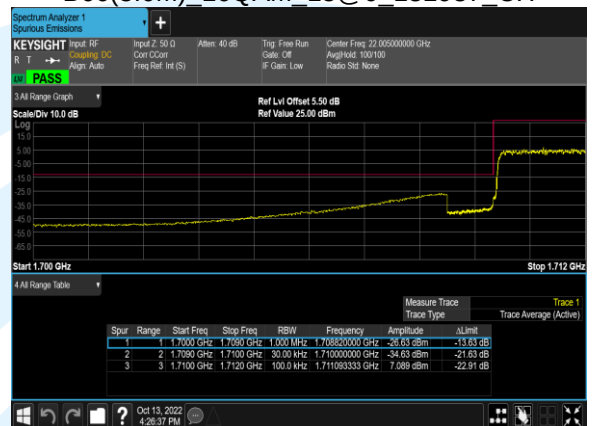
B66(3.0M) QPSK 15@0 132657 CH
