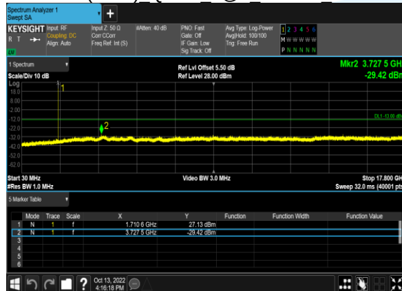
B66(1.4M) QPSK 1@0 131979 CH
