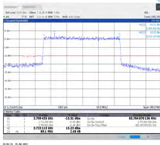
1-N78-3700-3800--30-90-H-1-DFT-QPSK-Outer_Full -240@0-Ant0-85.785-89.100-≤90-PASS
