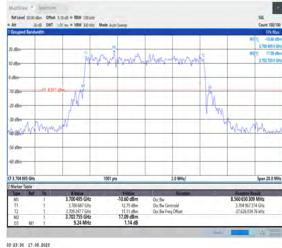
1-N78-3700-3800-PC1-30-10-L-2-DFT-PI2BPSK-Outer_Full-24@0-Ant0-8.561-9.240-≤10-PASS
