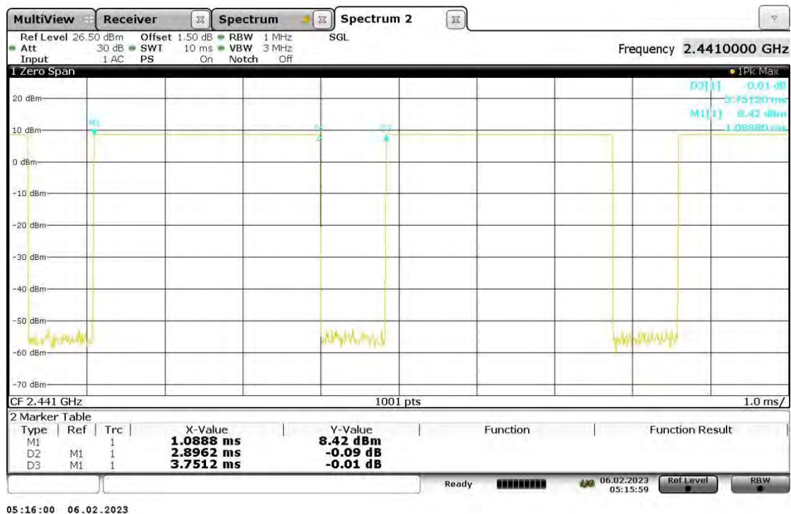
DH5_Ant1_2441
