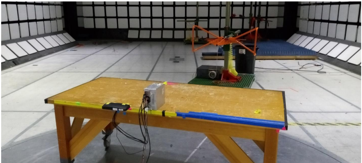
30MHz – 1 GHz, Y Axis
