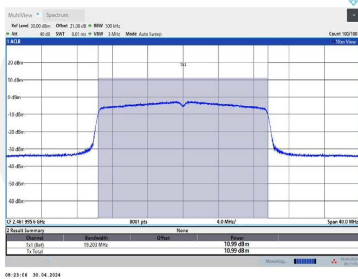
11AX20MIMO_Ant2_2462
