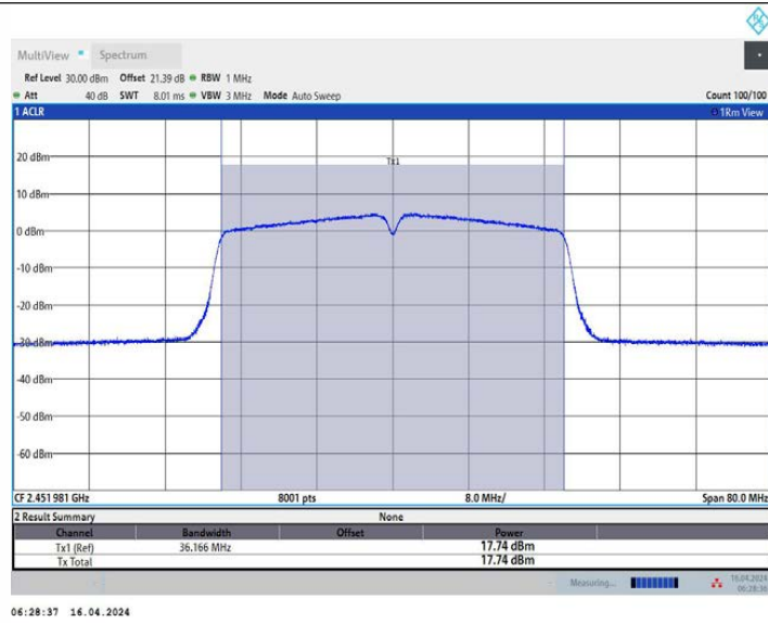
11N40MIMO_Ant2_2452
