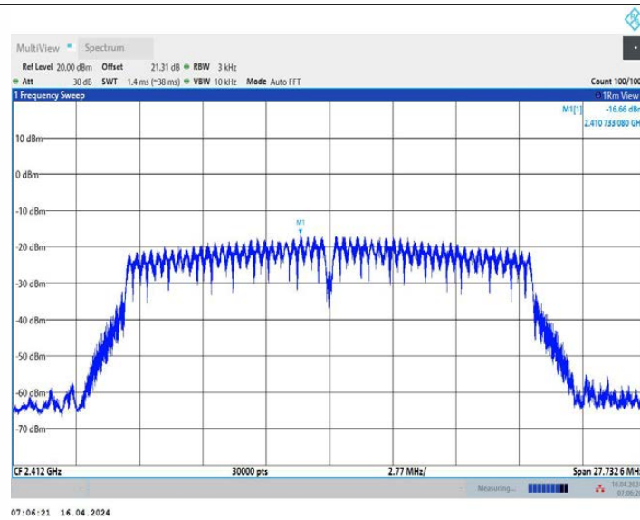
11N20MIMO_Ant2_2412
