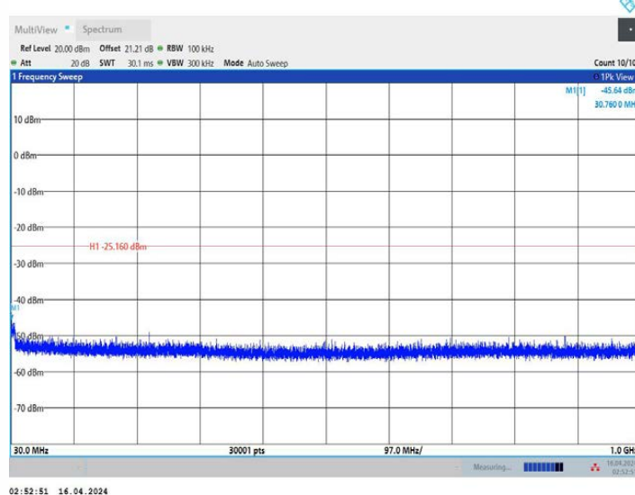
11G_Ant1_2412_30~1000
