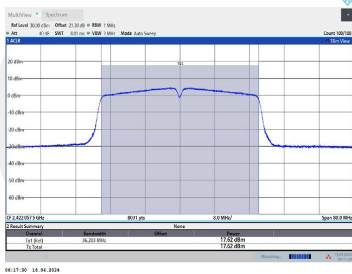
11N40MIMO_Ant2_2422
