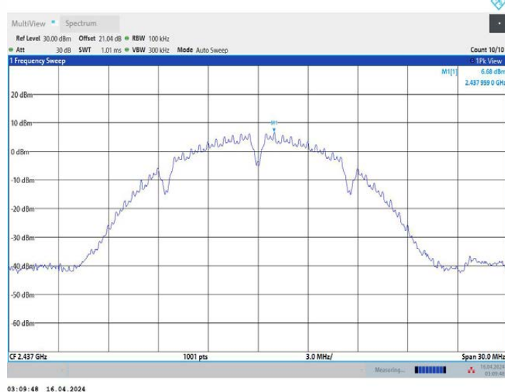
11B_Ant2_2437_0~Reference
