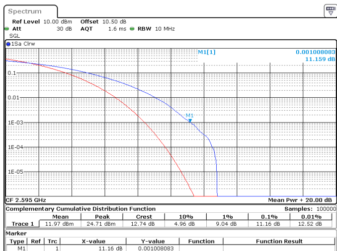
10MHz_30kHz_2595MHz_CP-OFDM 256 QAM_RB24@0 11.16 dB
