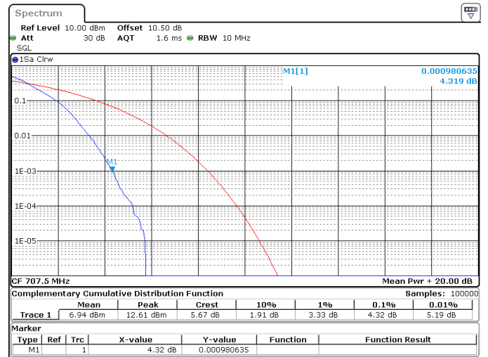
10MHz_15kHz_707.5MHz_DFT-s-OFDM PI/2 BPSK_RB50@0 4.32 dB
