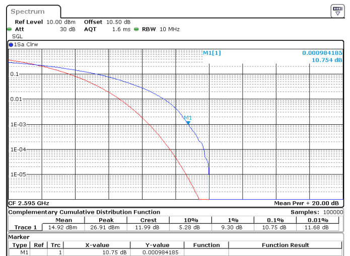
10MHz_30kHz_2595MHz_CP-OFDM 16 QAM_RB24@0 10.75 dB
