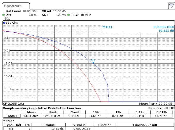
10MHz_30kHz_2355MHz_CP-OFDM 256 QAM_RB24@0 10.52 dB
