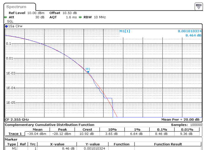
10MHz_30kHz_2355MHz_CP-OFDM 64 QAM_RB24@0 8.46 dB
