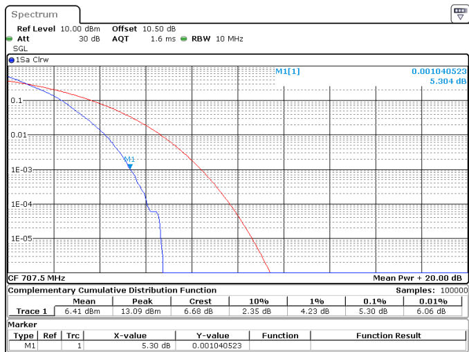
10MHz_15kHz_707.5MHz_DFT-s-OFDM QPSK_RB50@0 5.30 dB
