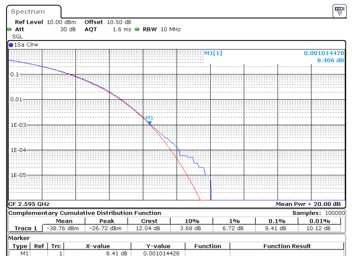
10MHz_30kHz_2595MHz_CP-OFDM 64 QAM_RB24@0 8.41 dB
