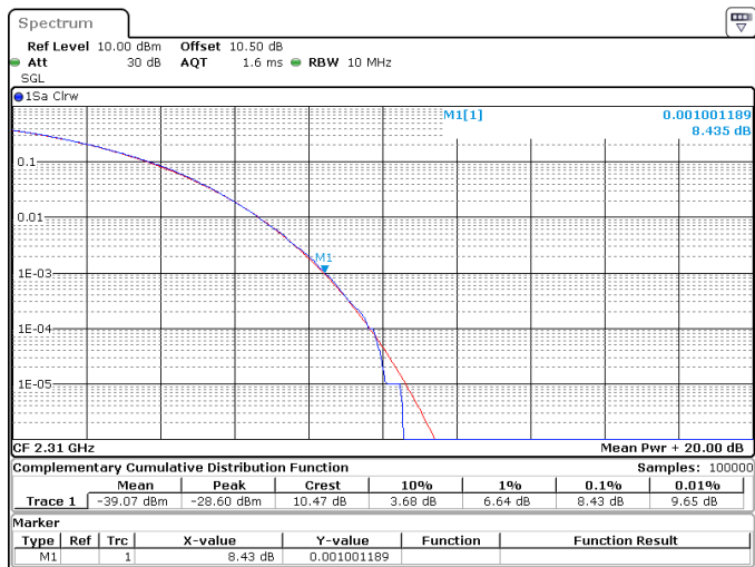
10MHz_30kHz_2310MHz_DFT-s-OFDM QPSK_RB24@0 8.43 dB
