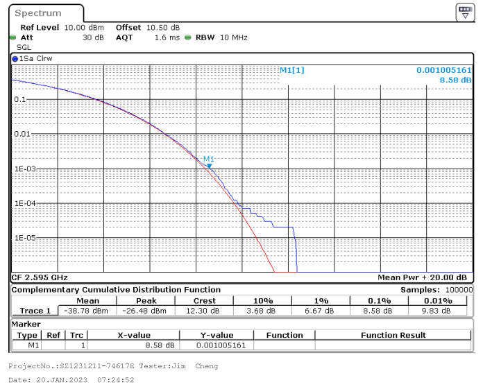
10MHz_30kHz_2595MHz_DFT-s-OFDM 16 QAM_RB24@0 8.58 dB
