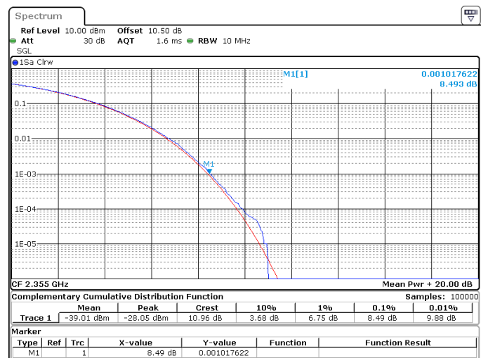
10MHz_30kHz_2355MHz_CP-OFDM 16 QAM_RB24@0 8.49 dB
