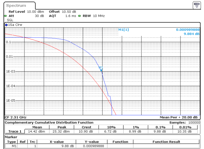
10MHz_30kHz_2310MHz_DFT-s-OFDM PI/2 BPSK_RB24@0 9.88 dB
