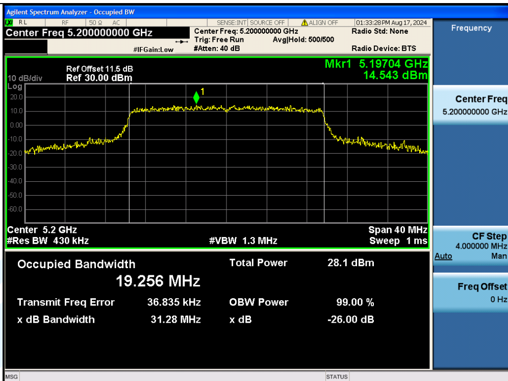
11AX20MIMO-Ant2-5200
