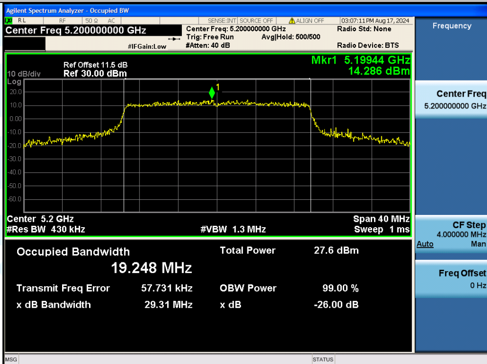
11AX20MIMO-Ant1-5240
