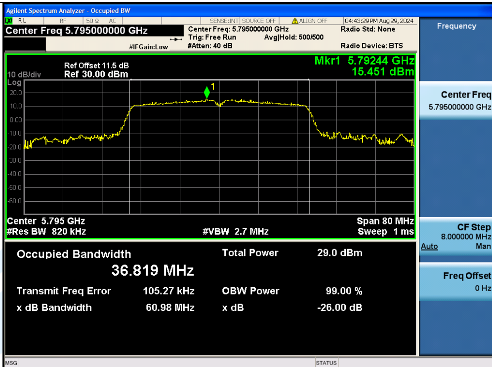
11N40MIMO-Ant2-5795
