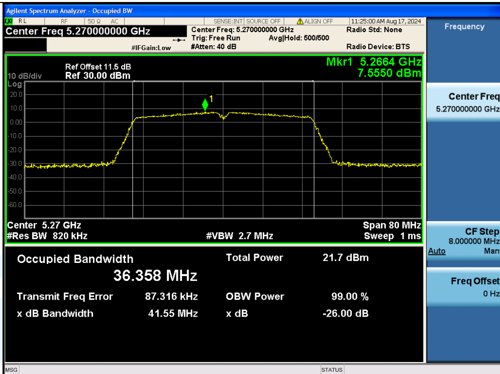
11N40MIMO-Ant2-5270
