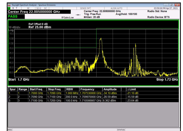
N66(20M)_DFT-s-OFDM_QPSK_Edge_1RB_L eft_Low_CH
