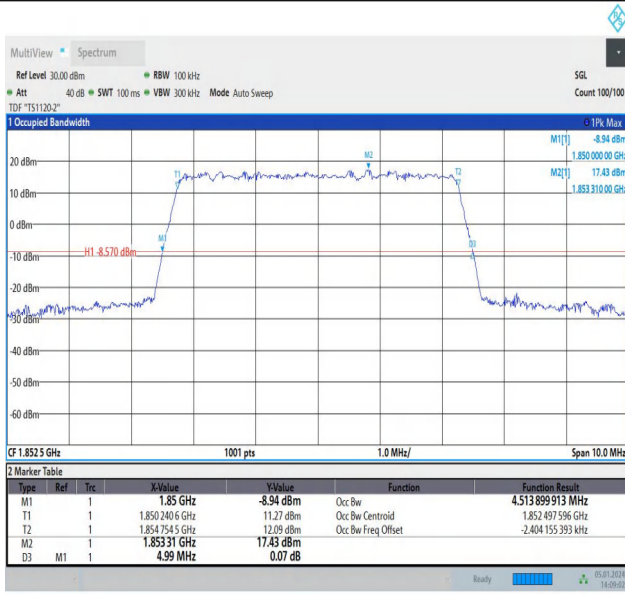
Band2-5MHz-QPSK-18625-25RB#0-PASS
