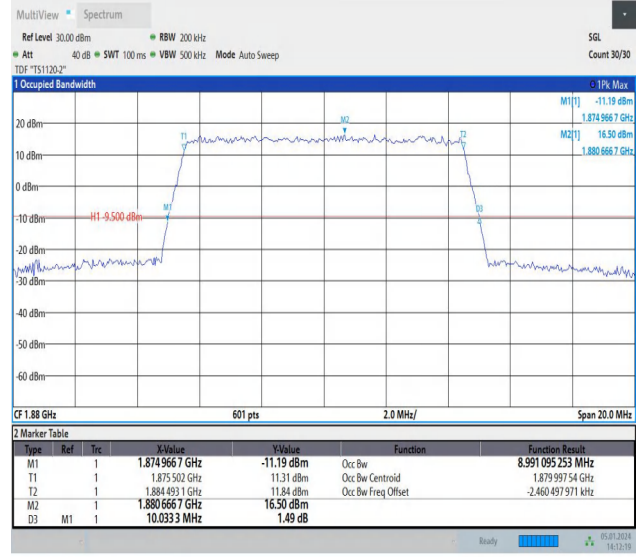
Band2-10MHz-16QAM-18900-50RB#0-PASS
