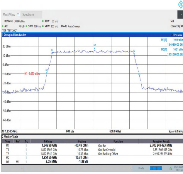
Band2-3MHz-QPSK-18615-15RB#0-PASS
