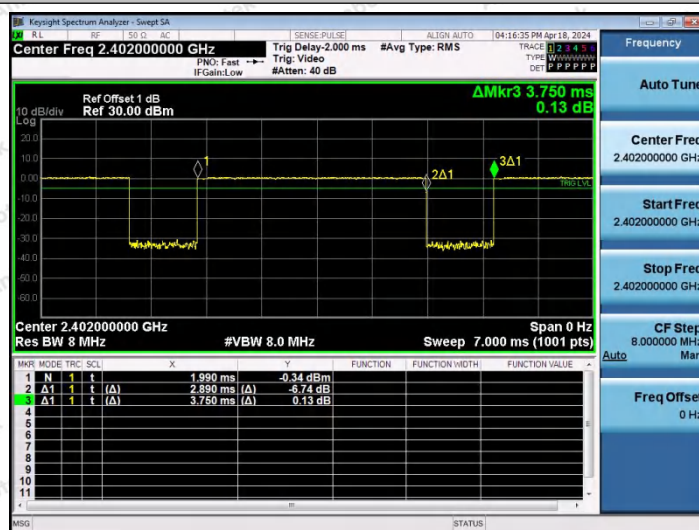
NTNV-2DH5-Ant1-2402
