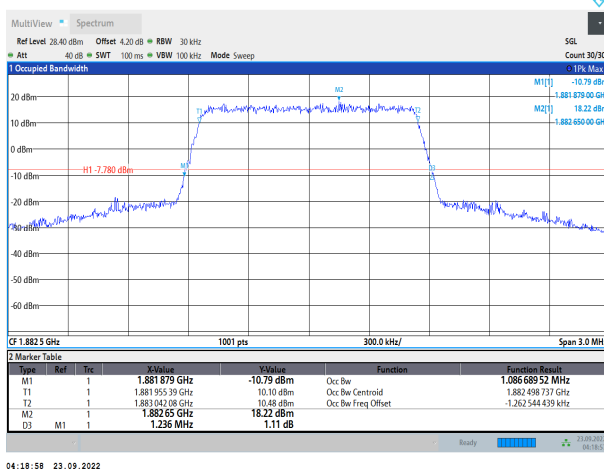
Band25-1.4MHz-QPSK-26365-6RB#0
