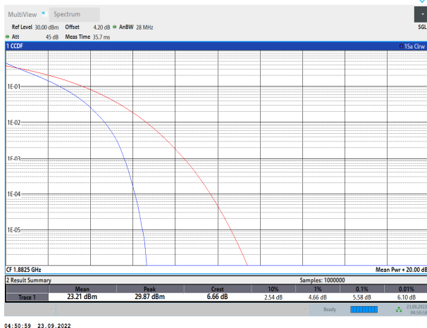
Band25-20MHz-QPSK-26365-100RB#0
