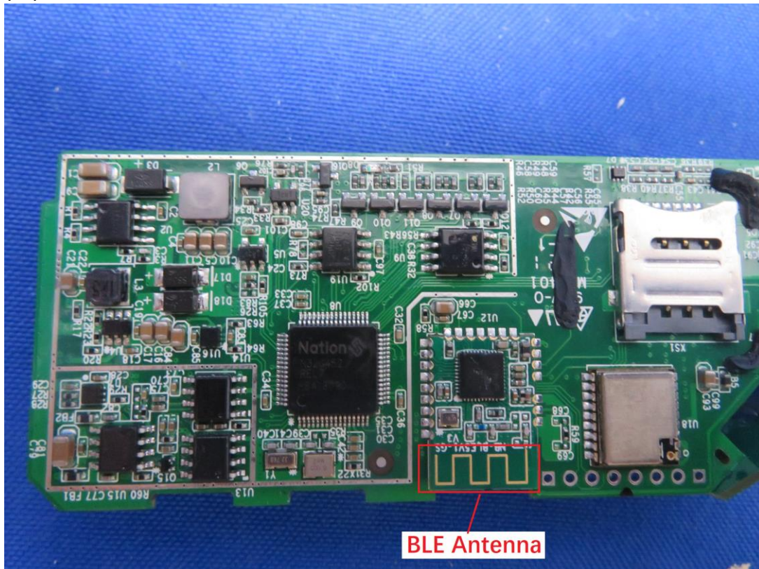
(12) EUT Photo
