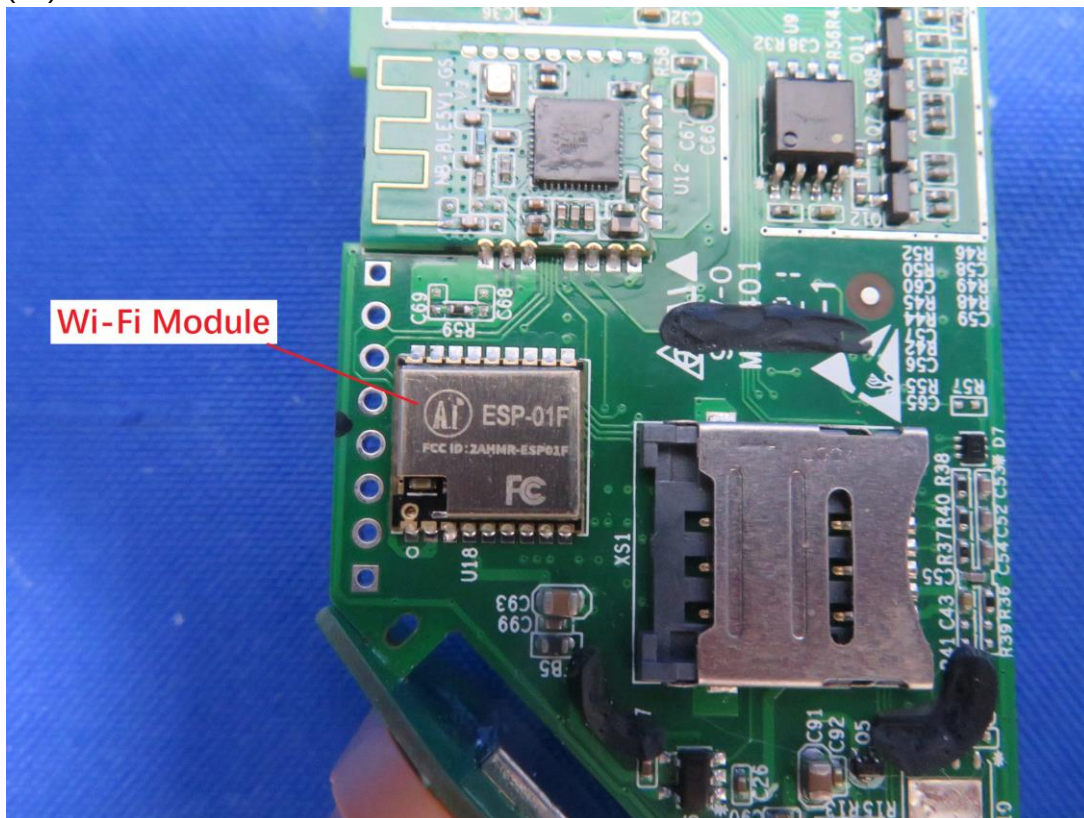
(12) EUT Photo
