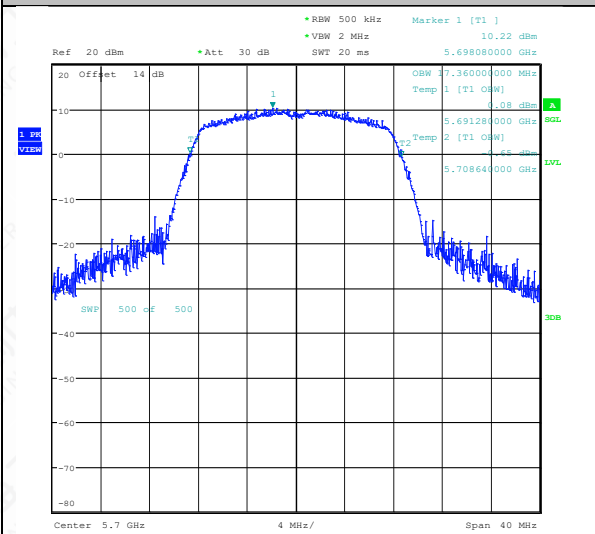
11A-Ant1-5700
