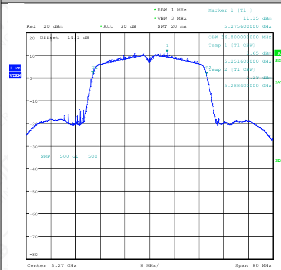
11N40SISO-Ant1-5270
