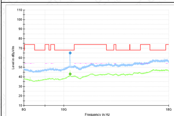
RSE-11N-CH36-8GHz-18GHz
