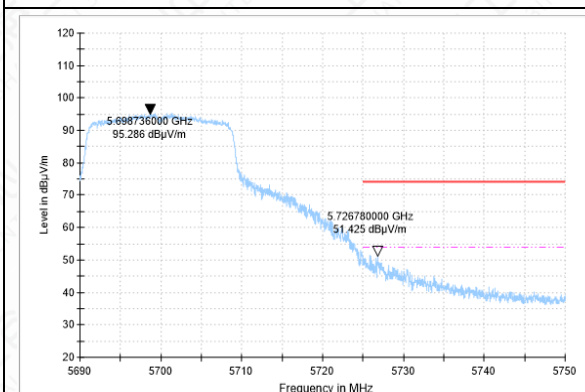
BANDEGE-11AC-CH140-AV
