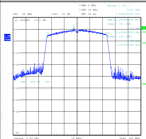
11AC80SISO-Ant1-5530
