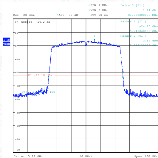
11AC80SISO-Ant1-5290
