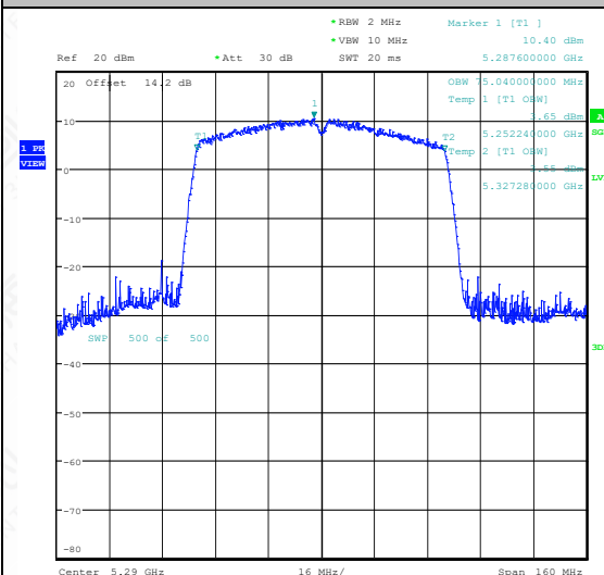
11AC80SISO-Ant1-5290
