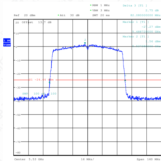
11AC80SISO-Ant1-5530
