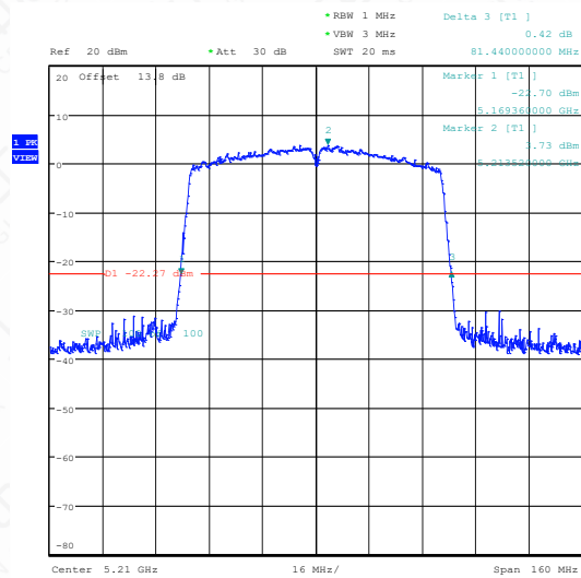
11AC80SISO-Ant1-5210
