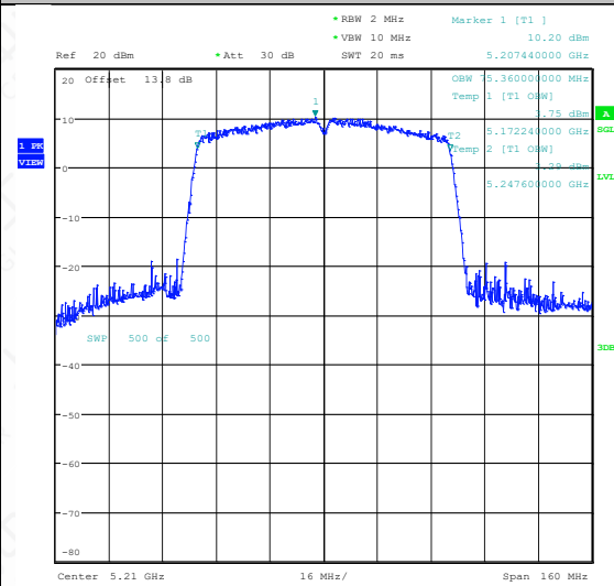
11AC80SISO-Ant1-5210
