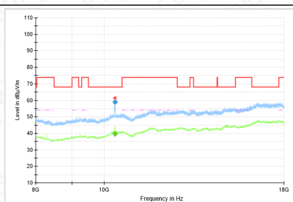
RSE-11AC-CH36-8GHz-18GHz
