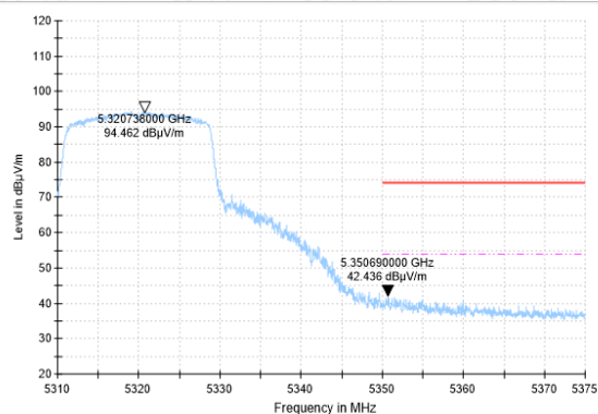
BANDEGE-11AC-CH64-AV
