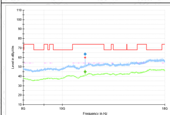
RSE-11A-CH140-8GHz-18GHz
