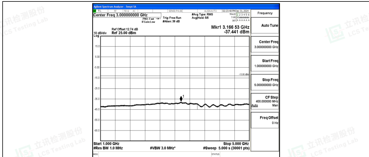
Band5-5MHz-QPSK-20425-1-0-Low-1000-5000--37.44-PASS
