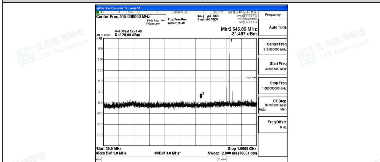
Band5-5MHz-QPSK-20425-1-0-Low-30-1000--31.49-PASS
