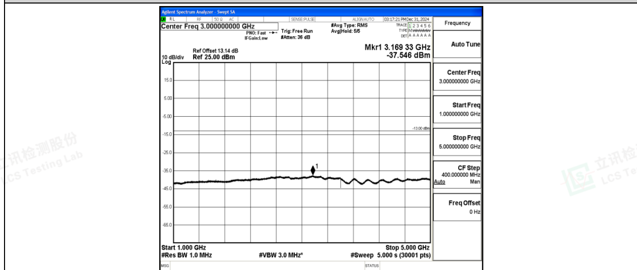
Band5-10MHz-QPSK-20525-1-0-Low-1000-5000--37.55-PASS
