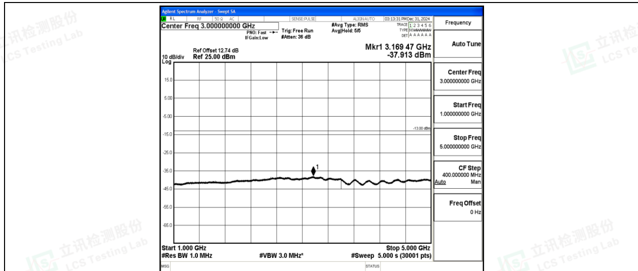
Band5-10MHz-QPSK-20450-1-0-Low-1000-5000--37.91-PASS
