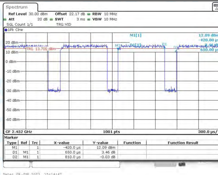
11N40-CDD_Ant2_2452
