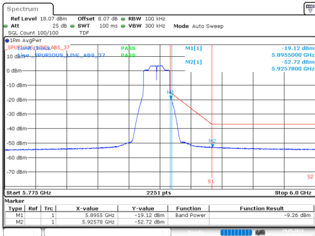
BE-NR-HIGH, MIMO-A, 802.11ax/be20-MCS0, Ch177
