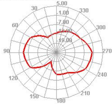
5300.000MHz H
