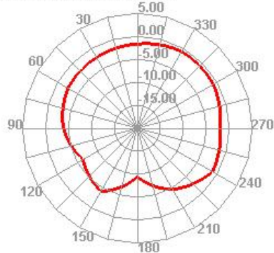
5300.000MHz E2
