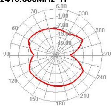
2410.000MHz H
