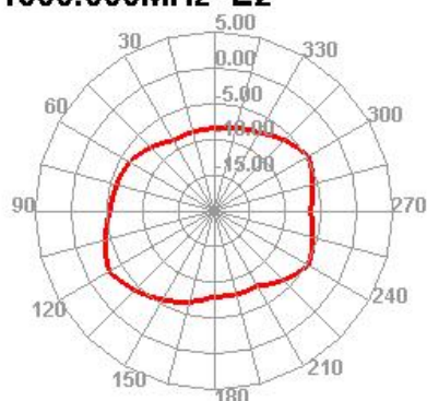
1500.000MHz E2
