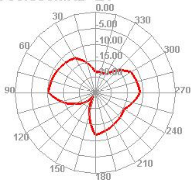
700.000MHz E1
