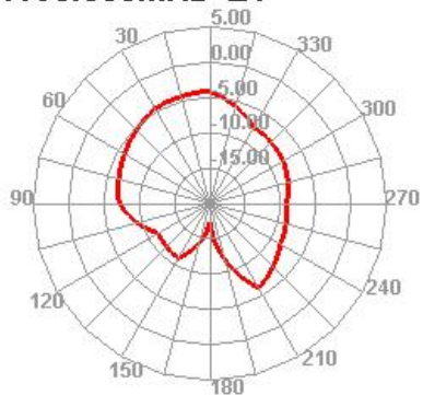
1690.000MHz E1
