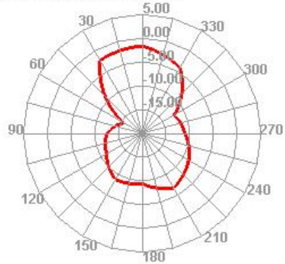
5300.000MHz E1
