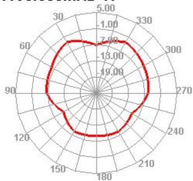
1690.000MHz H
