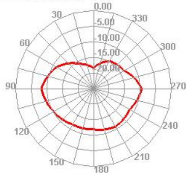
700.000MHz E2
