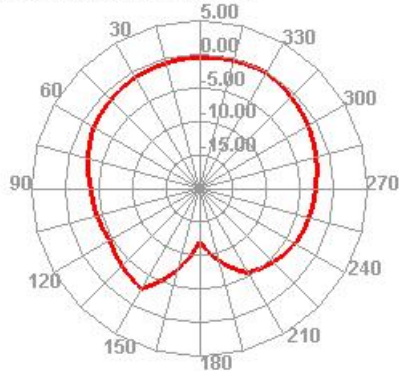
5100.000MHz E2
