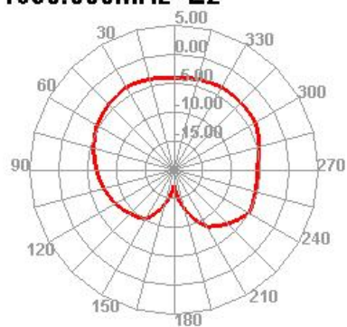
1690.000MHz E2
