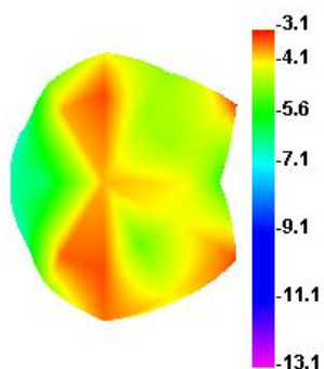
1690.000MHz
