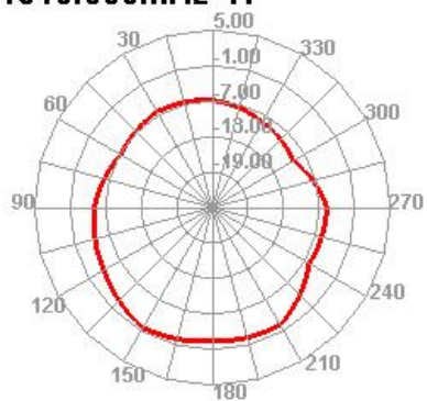
1510.000MHz H
