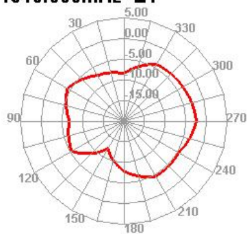
1510.000MHz E1
