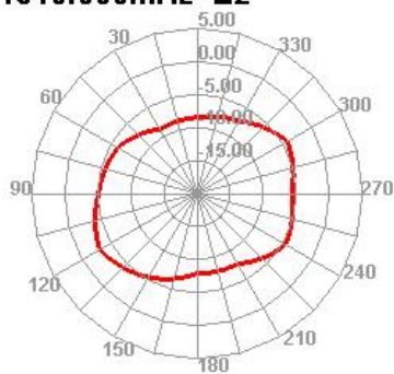
1510.000MHz E2
