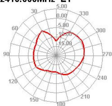
2410.000MHz E1
