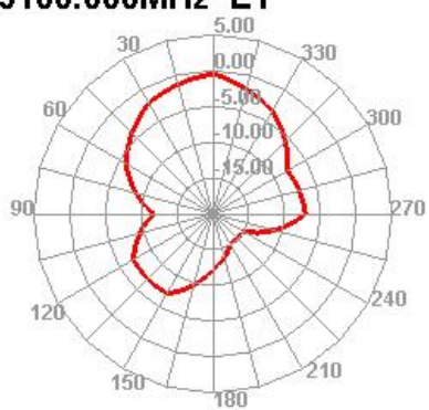
5100.000MHz E1
