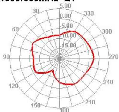
1500.000MHz E1
