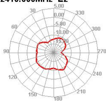
2410.000MHz E2
