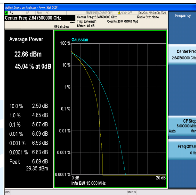
Band41(2555-2655)-15MHz-QPSK-41165-75RB#0-PASS
