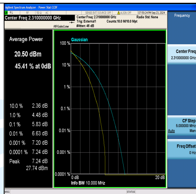
Band40(2305-2315)-10MHz-QPSK-38750-50RB#0-PASS
