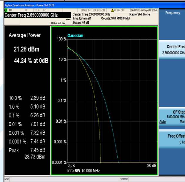
Band41(2555-2655)-10MHz-16QAM-41190-50RB#0-PASS
