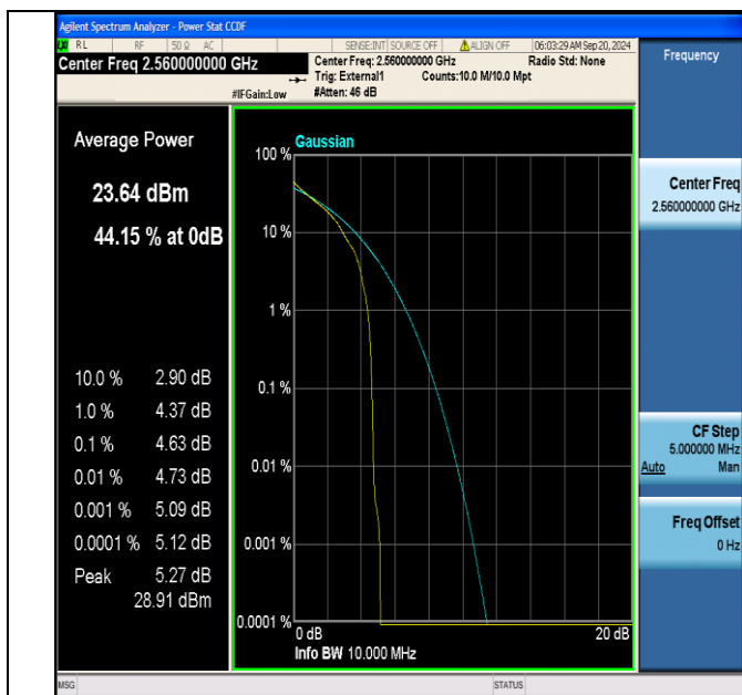
Band41(2555-2655)-10MHz-QPSK-40290-1RB#0-PASS
