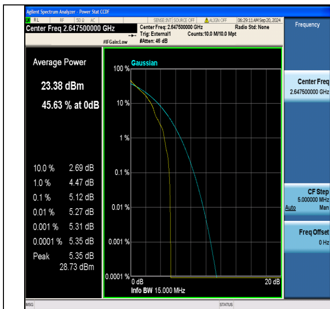
Band41(2555-2655)-15MHz-QPSK-41165-1RB#0-PASS
