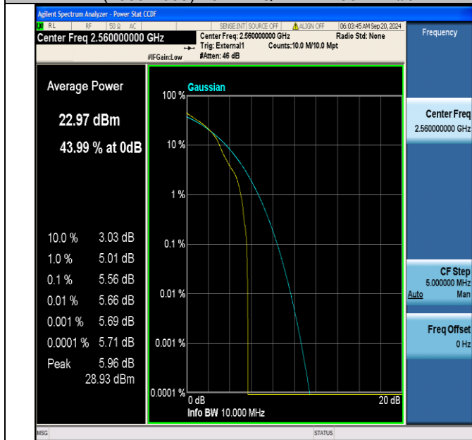
Band41(2555-2655)-10MHz-16QAM-40290-1RB#0-PASS
