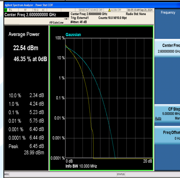
Band41(2555-2655)-10MHz-QPSK-40690-50RB#0-PASS
