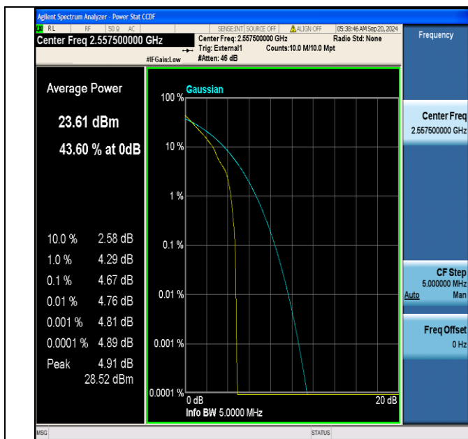
Band41(2555-2655)-5MHz-QPSK-40265-1RB#0-PASS
