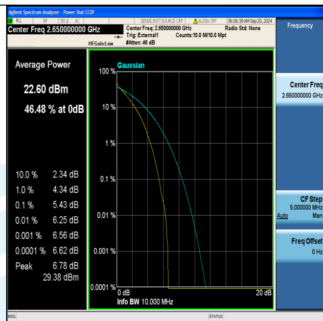
Band41(2555-2655)-10MHz-QPSK-41190-50RB#0-PASS
