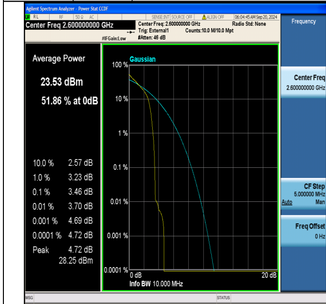
Band41(2555-2655)-10MHz-QPSK-40690-1RB#0-PASS
