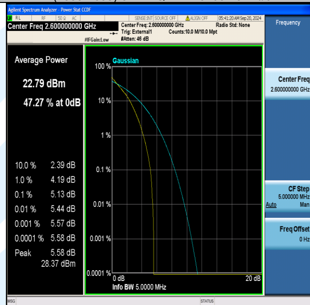
Band41(2555-2655)-5MHz-QPSK-40690-25RB#0-PASS
