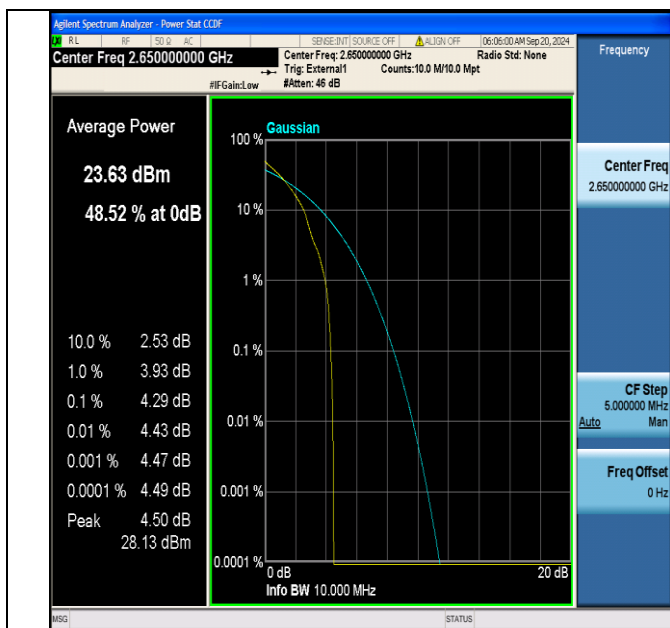
Band41(2555-2655)-10MHz-QPSK-41190-1RB#0-PASS
