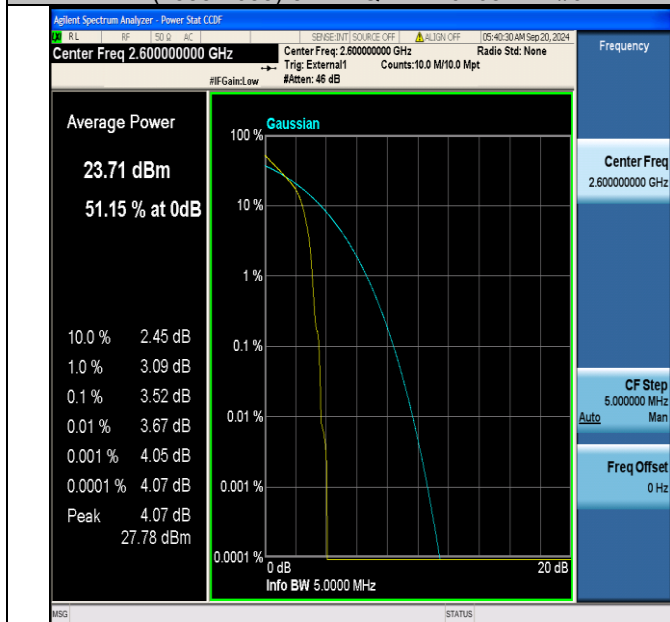
Band41(2555-2655)-5MHz-QPSK-40690-1RB#0-PASS
