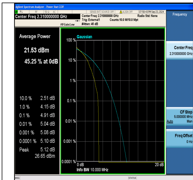
Band40(2305-2315)-10MHz-QPSK-38750-1RB#0-PASS
