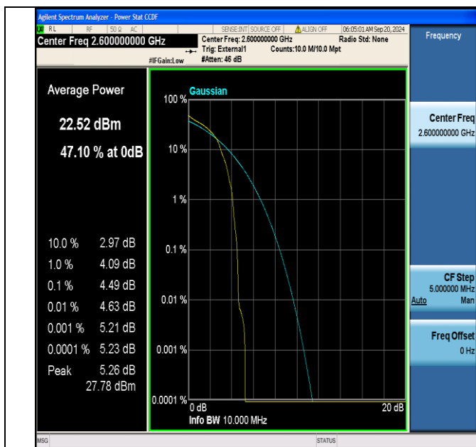
Band41(2555-2655)-10MHz-16QAM-40690-1RB#0-PASS
