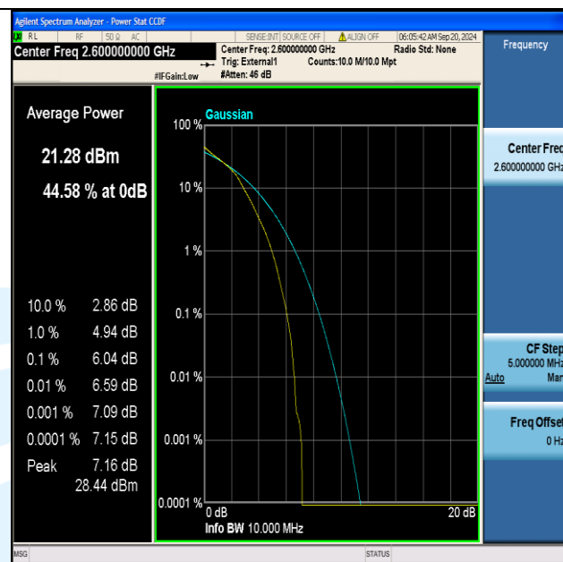
Band41(2555-2655)-10MHz-16QAM-40690-50RB#0-PASS
