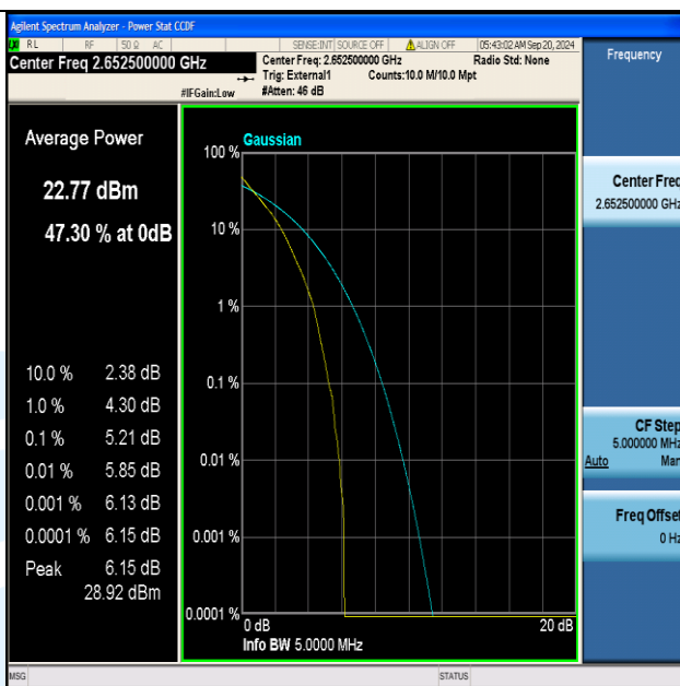
Band41(2555-2655)-5MHz-QPSK-41215-25RB#0-PASS
