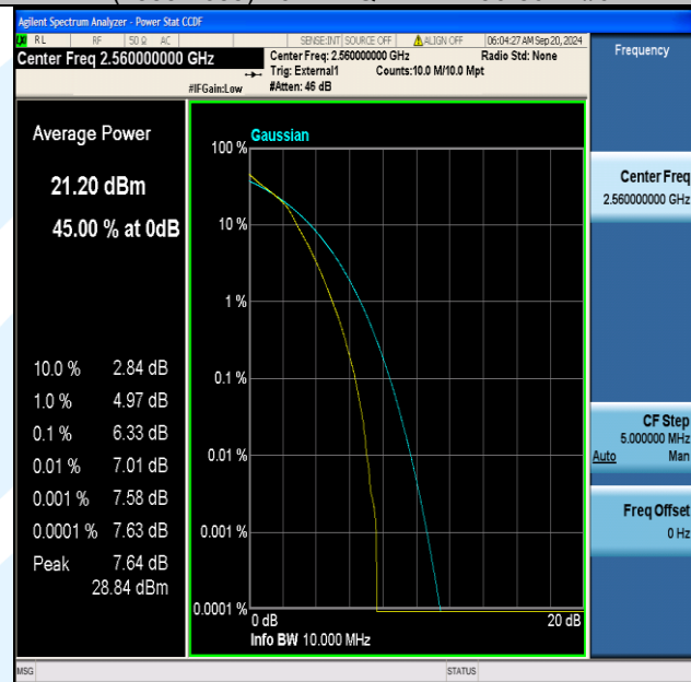
Band41(2555-2655)-10MHz-16QAM-40290-50RB#0-PASS
