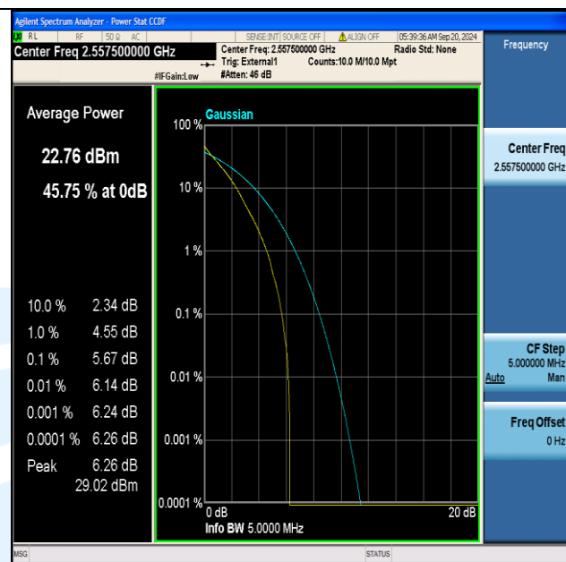
Band41(2555-2655)-5MHz-QPSK-40265-25RB#0-PASS
