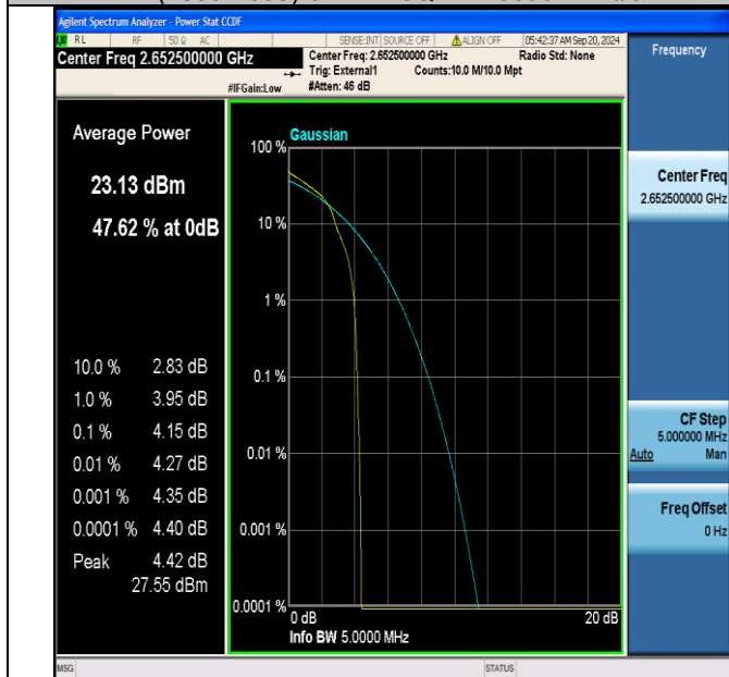
Band41(2555-2655)-5MHz-16QAM-41215-1RB#0-PASS
