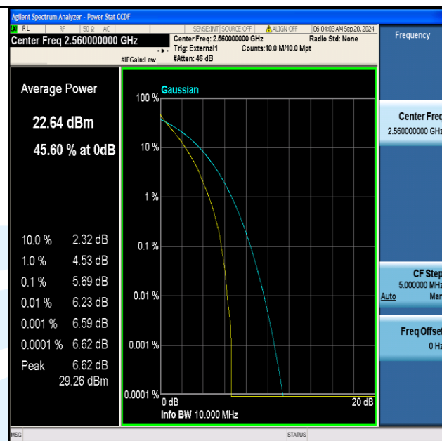
Band41(2555-2655)-10MHz-QPSK-40290-50RB#0-PASS
