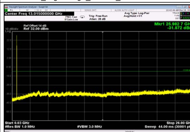
FDD17_HighRange_10MHz_30MHz~26GHz
