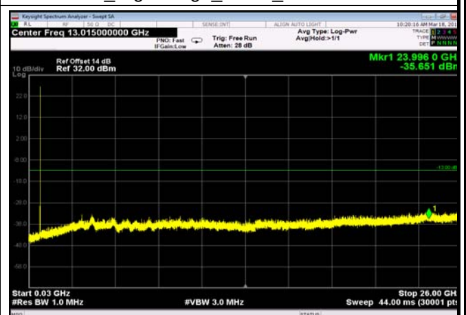
FDD17_HighRange_5MHz_30MHz~26GHz
