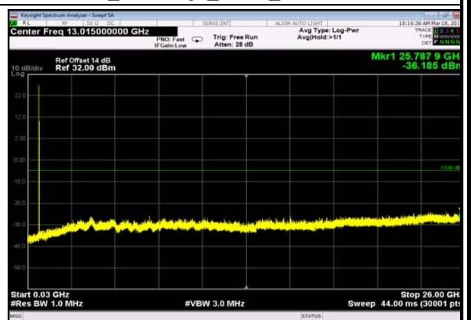
FDD13_HighRange_5MHz_30MHz~26GHz
