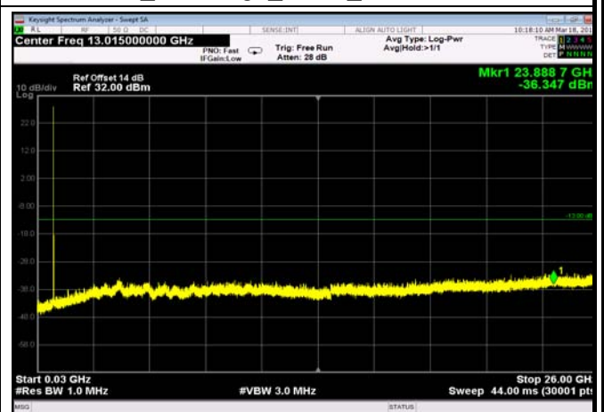
FDD17_HighRange_5MHz_30MHz~26GHz
