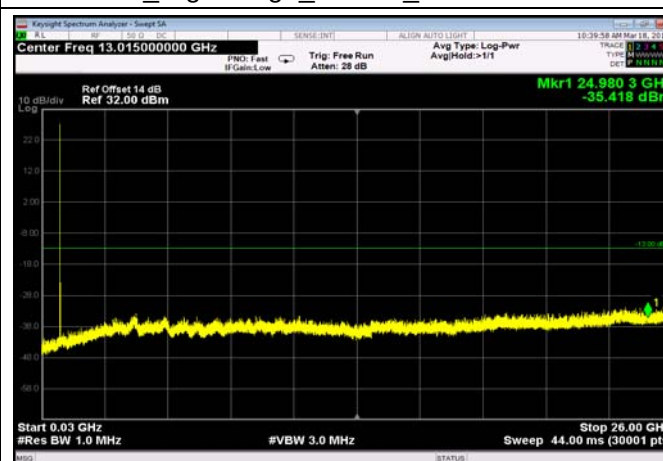
FDD13_HighRange_10MHz_30MHz~26GHz
