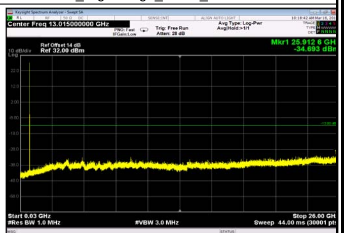
FDD13_HighRange_5MHz_30MHz~26GHz
