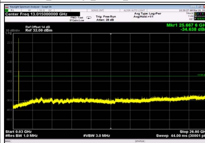
FDD17_HighRange_10MHz_30MHz~26GHz
