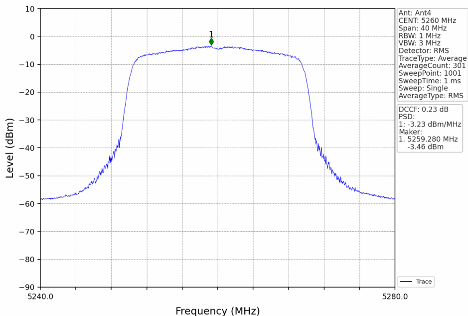
802.11ax(HEW20)_LCH_5260MHz_RU242_Left_Ant4_NTNV
