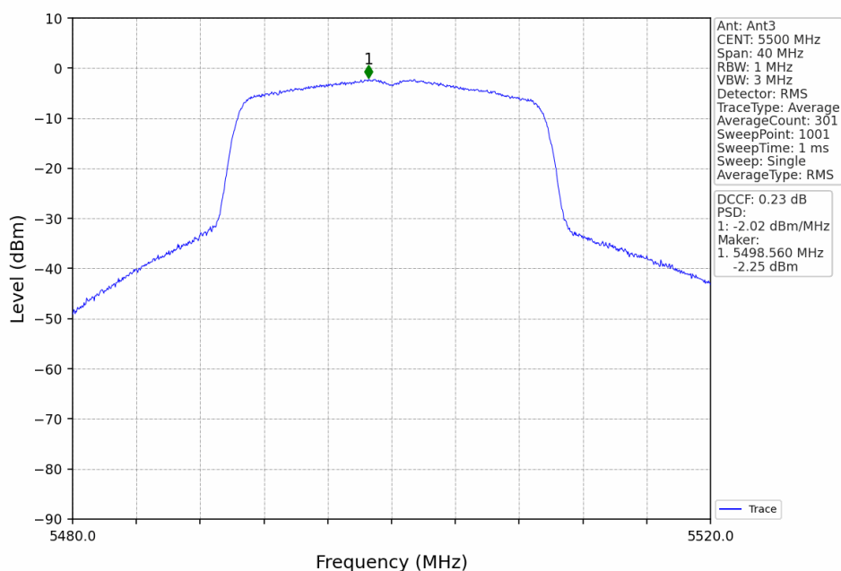
802.11ax(HEW20)_LCH_5500MHz_RU242_Left_Ant3_NTNV
