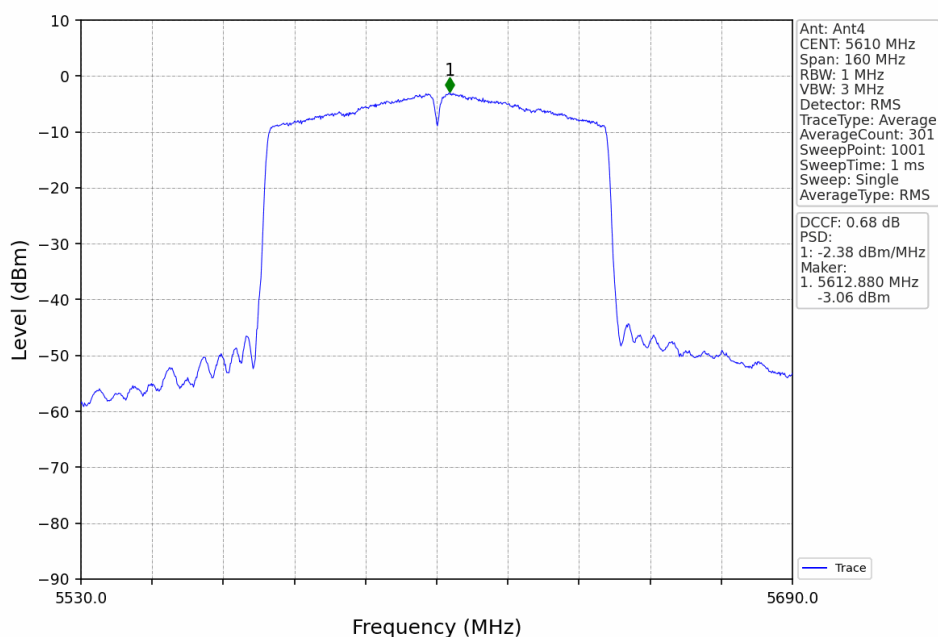
802.11ac(VHT80)_HCH_5610MHz_Ant4_NTNV
