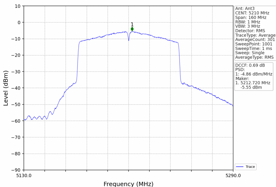
802.11ac(VHT80)_MCH_5210MHz_Ant3_NTNV
