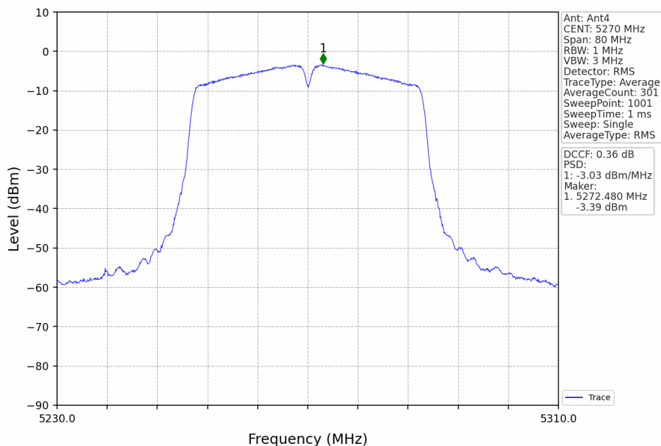
802.11ac(VHT40)_LCH_5270MHz_Ant4_NTNV
