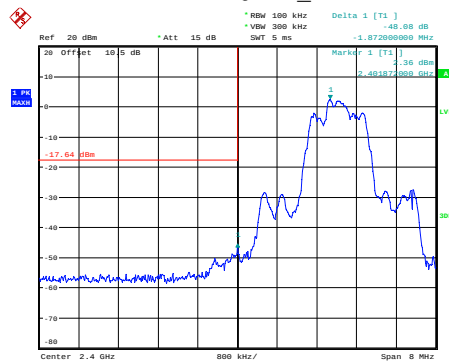
\pi/4 -DQPSK_Low
