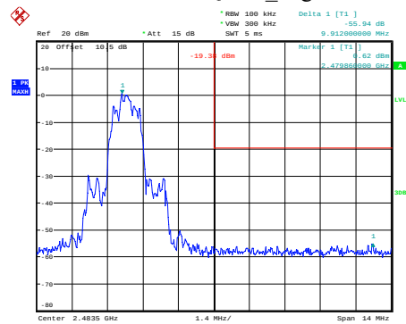
\pi/4 -DQPSK_High
