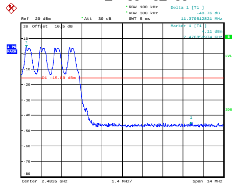
GFSK_Hopping_Upper
