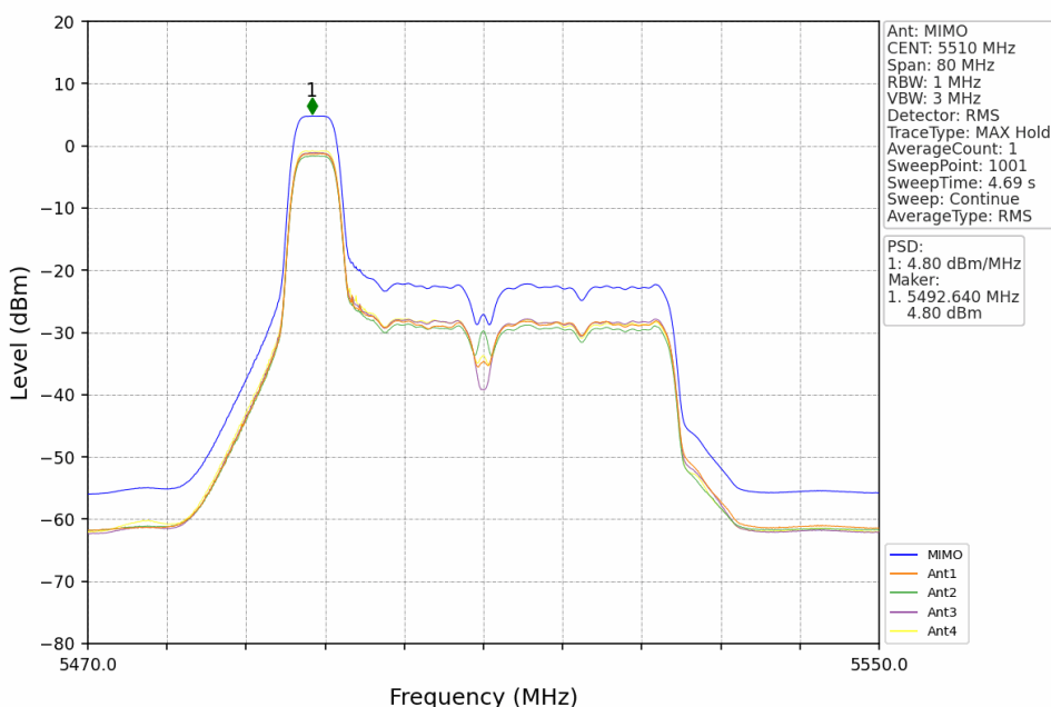
802.11be(EHT40)_LCH_5510MHz_RU52+26_Left_MIMO_NTNV
