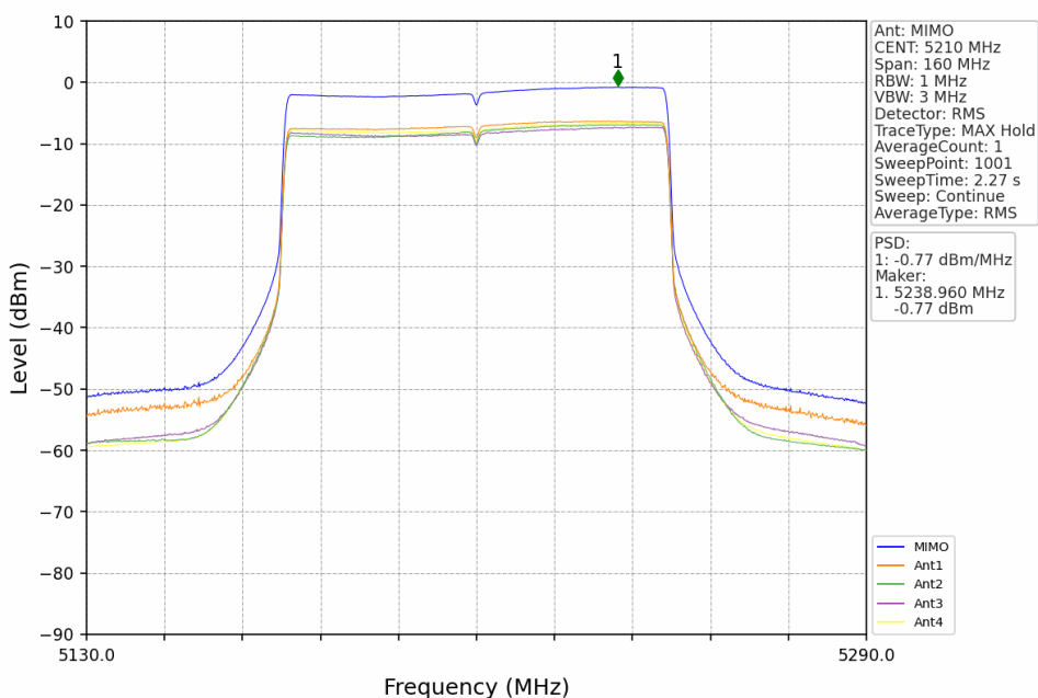
802.11ax(HEW80)_MCH_5210MHz_RU996_Left_MIMO_NTNV
