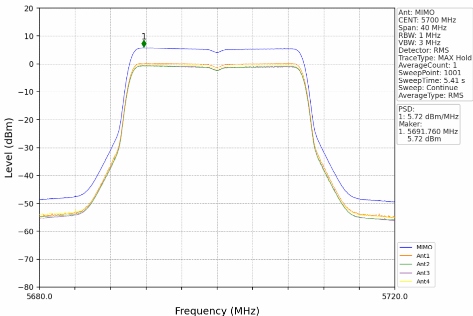
802.11be(EHT20)_HCH_5700MHz_RU242_Left_MIMO_NTNV
