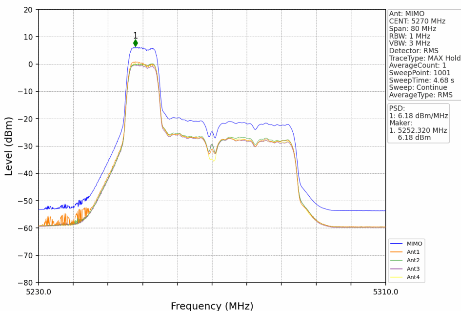
802.11be(EHT40)_LCH_5270MHz_RU52+26_Left_MIMO_NTNV
