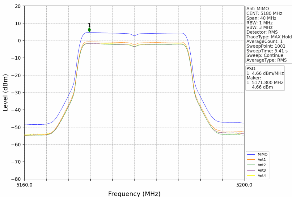
802.11be(EHT20)_LCH_5180MHz_RU242_Left_MIMO_NTNV
