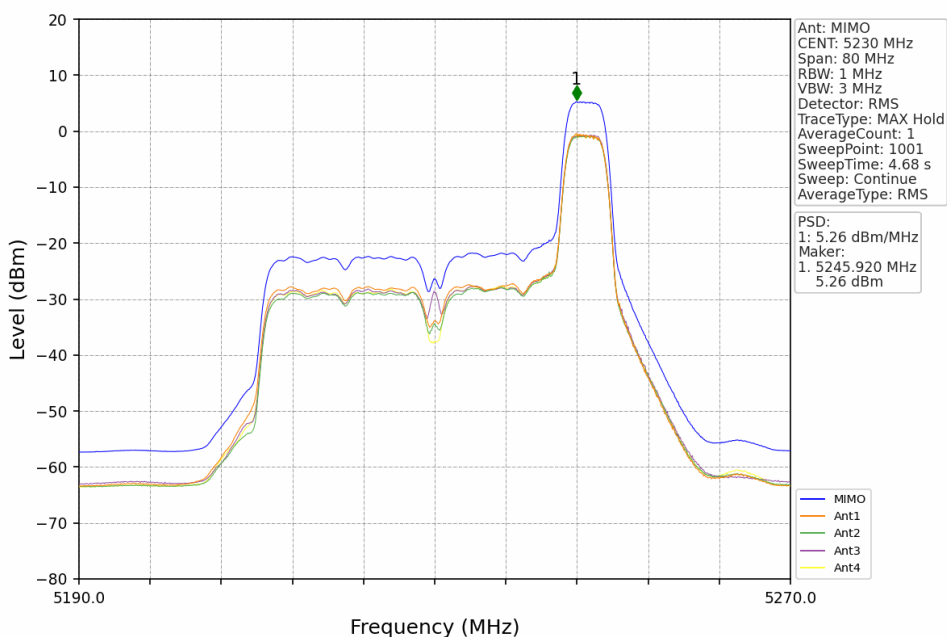
802.11be(EHT40)_HCH_5230MHz_RU52_Right_MIMO_NTNV
