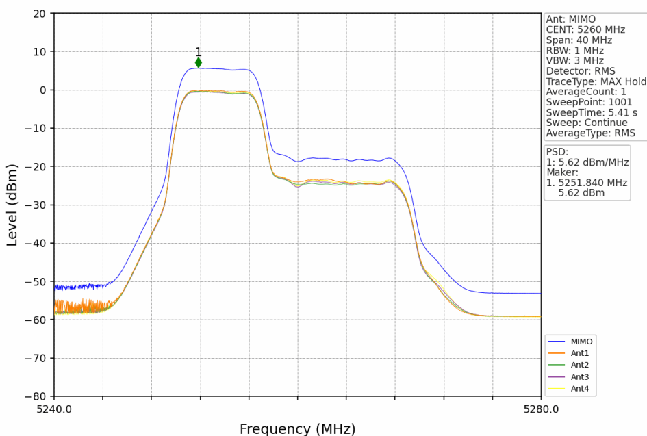
802.11be(EHT20)_LCH_5260MHz_RU52+26_Left_MIMO_NTNV
