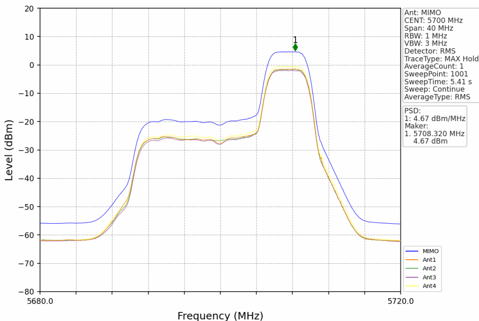
802.11be(EHT20)_HCH_5700MHz_RU52_Right_MIMO_NTNV
