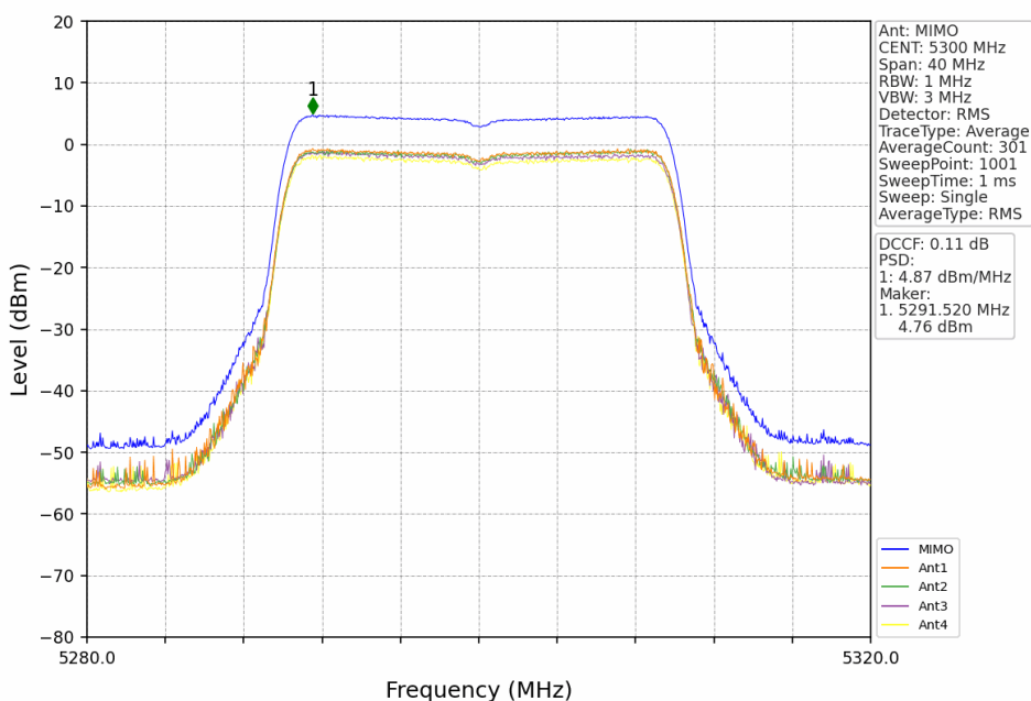
802.11be(EHT20)_MCH_5300MHz_RU242_Left_MIMO_NTNV
