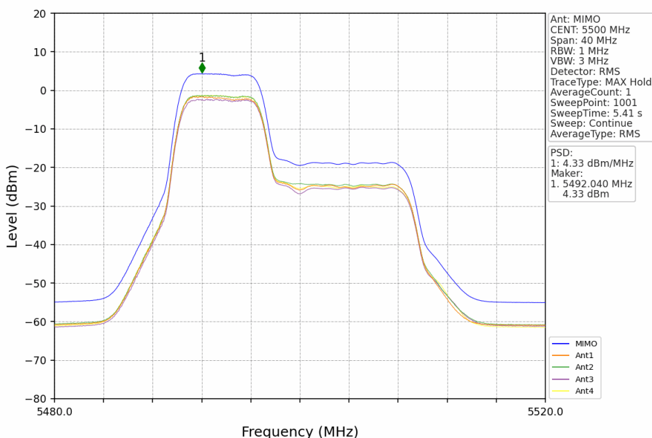
802.11be(EHT20)_LCH_5500MHz_RU242_Left_MIMO_NTNV
