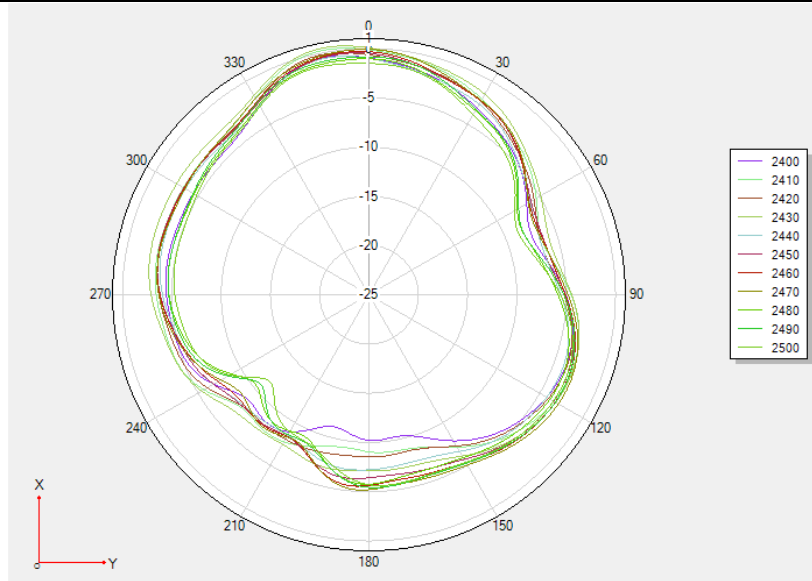
2400MHz 3D 放类似图 Z 轴朝上
