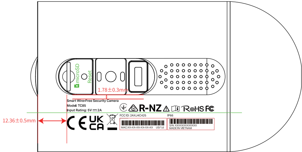
尺寸图
