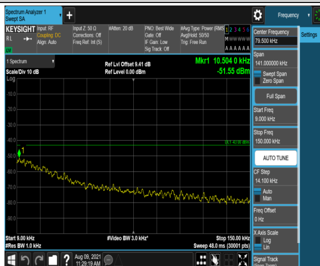
Band25-3MHz-QPSK-26365-1-0-Low-0.009-0.15--51.55-PASS
