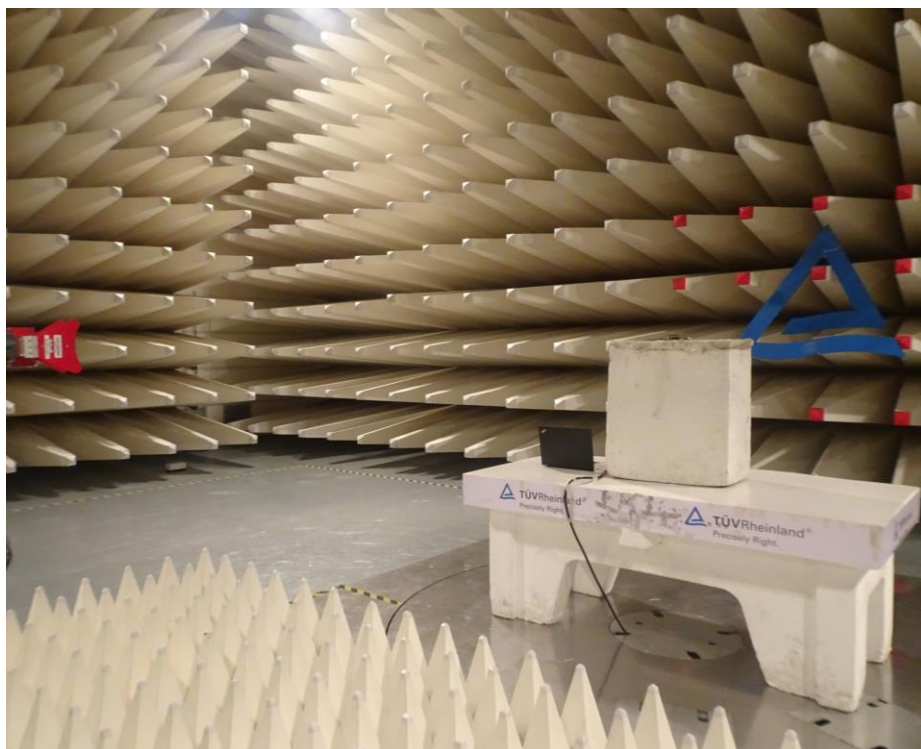
Test Setup: 18GHz – 26.5GHz
