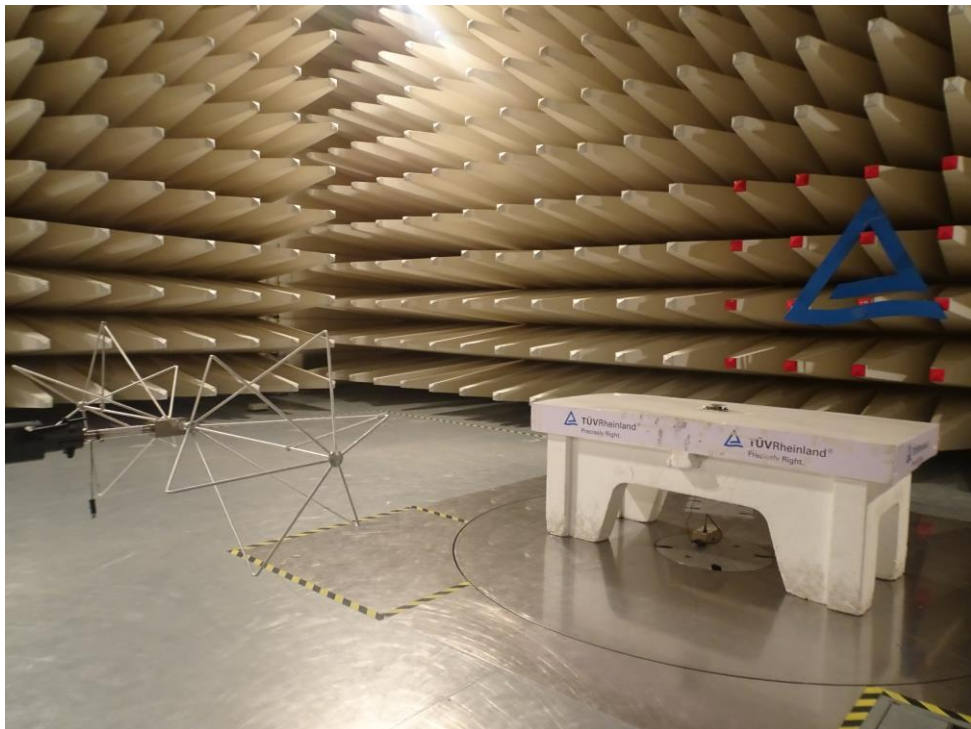
Test Setup: 30MHz-200MHz
