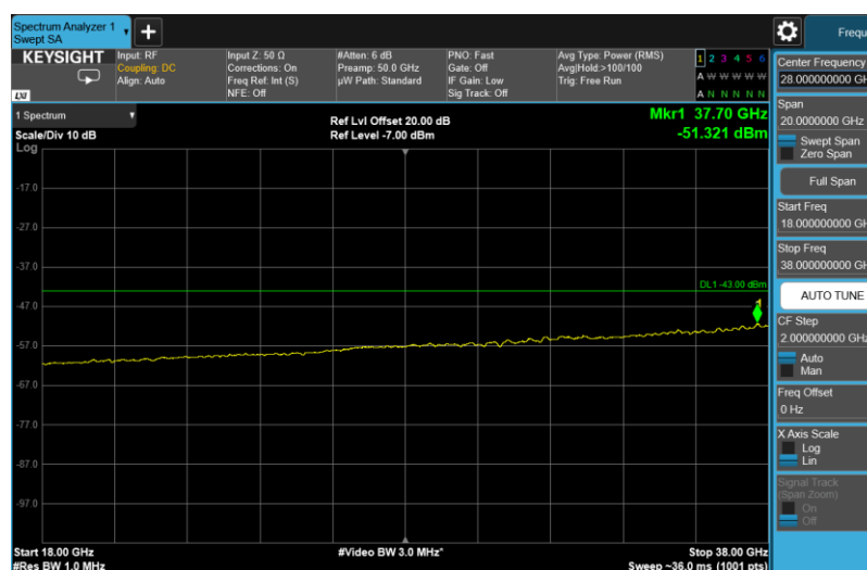
Channel: TOP, Modulation: QPSK, BW=20MHz, Range: 18GHz - 38GHz
