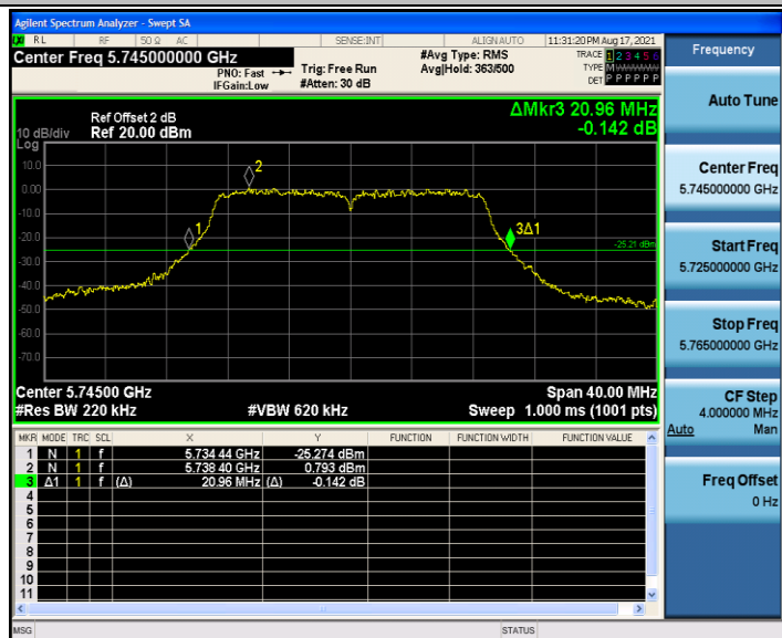
11AC20MIMO_Ant2_5745
